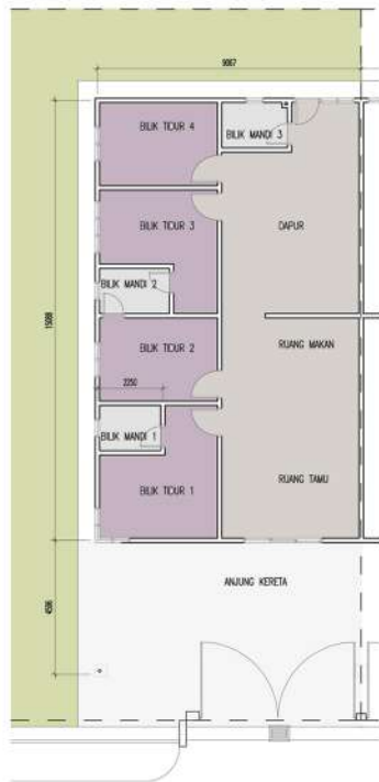
PELAN LANTAI
