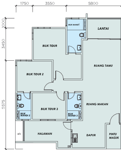
TYPE C Membrina : 1,465 sq. ft. 3 Bilik Tidur + 3 Bilik Mandi
