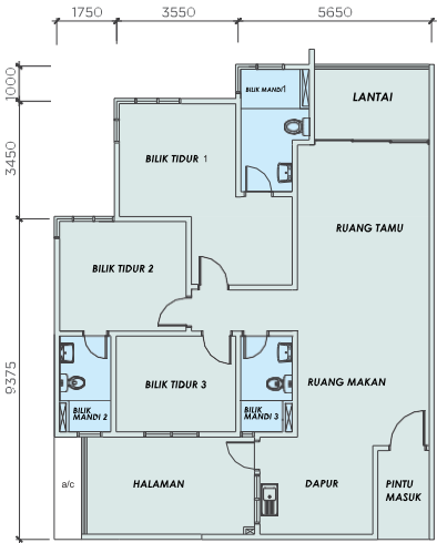
TYPE A Membrina : 1,472 sq. ft. 3 Bilik Tidur + 3 Bilik Mandi
