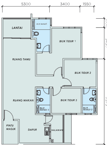
TYPE D Membrina : 1,283 sq. ft. 3 Bilik Tidur + 3 Bilik Mandi
