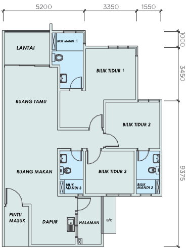
TYPE B Membrina : 1,253 sq. ft. 3 Bilik Tidur + 3 Bilik Mandi
