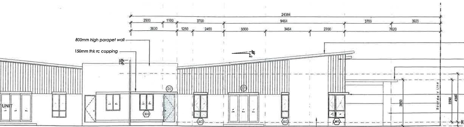
PANDANGAN TEPI
