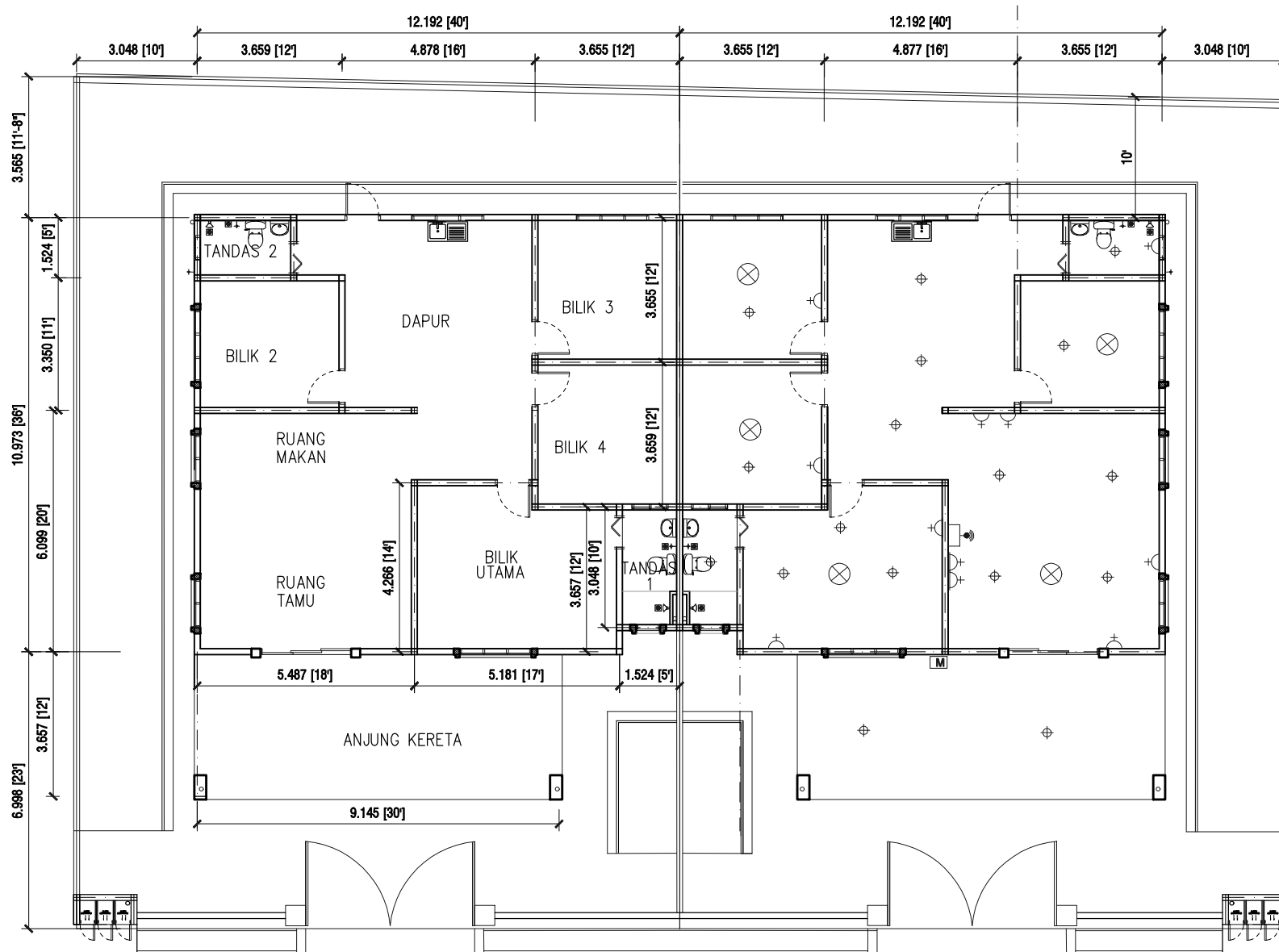
PELAN LANTAI (Rumah berbandung ( jenis 'C' - 40' X 36') - LOT 11249-LOT 11252
