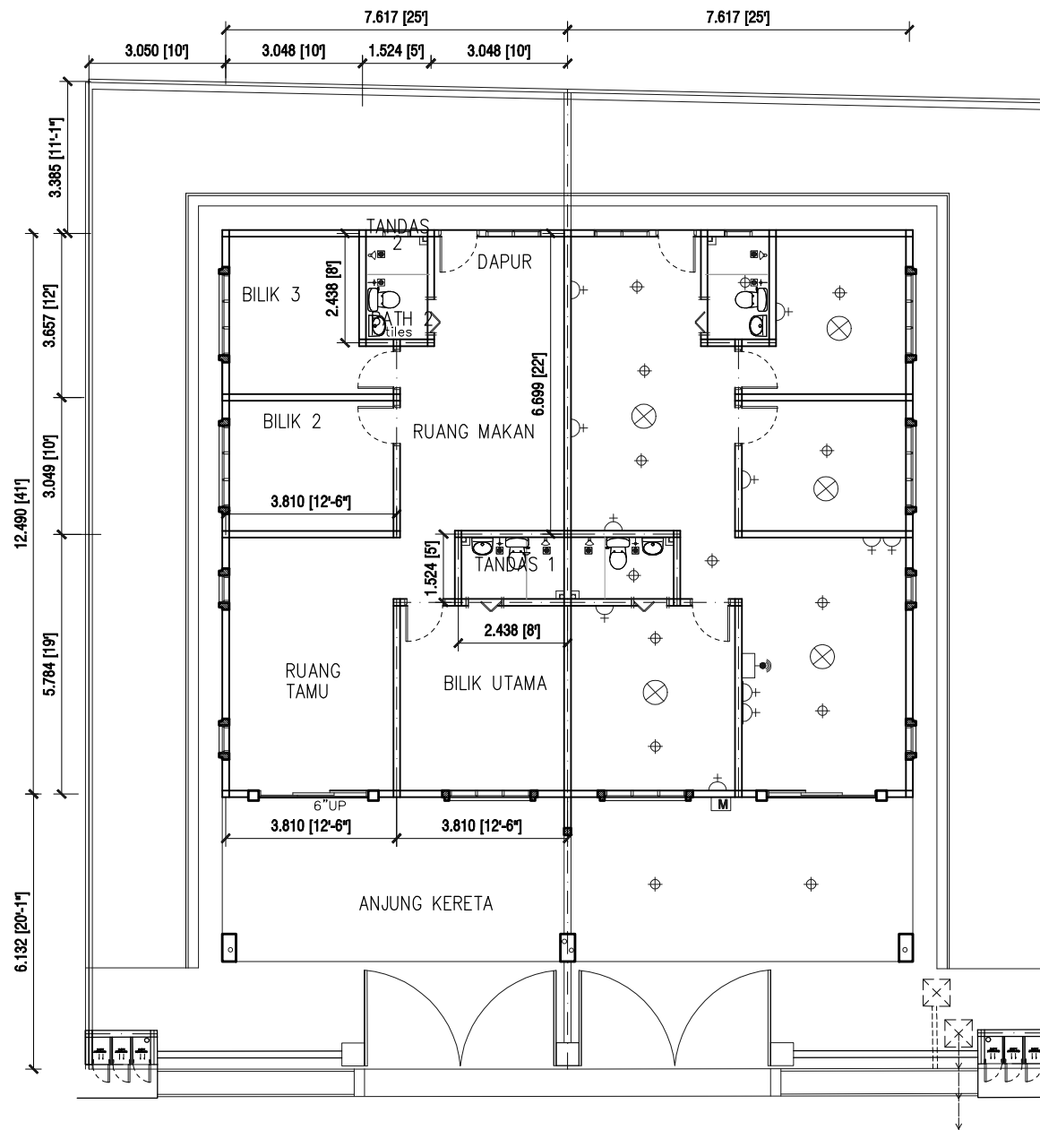
PELAN LANTAI (Rumah berbandung ( jenis 'B' - 25' X 41' ) - LOT 11245 - LOT 11248
