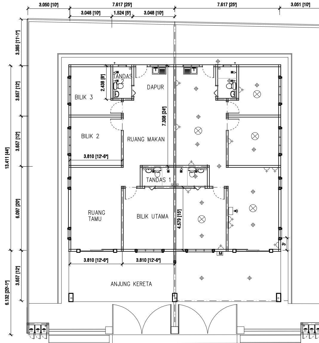
PELAN LANTAI (Rumah berbandung ( jenis 'A' - 25' X 44' )- LOT 11239 - LOT 11244
