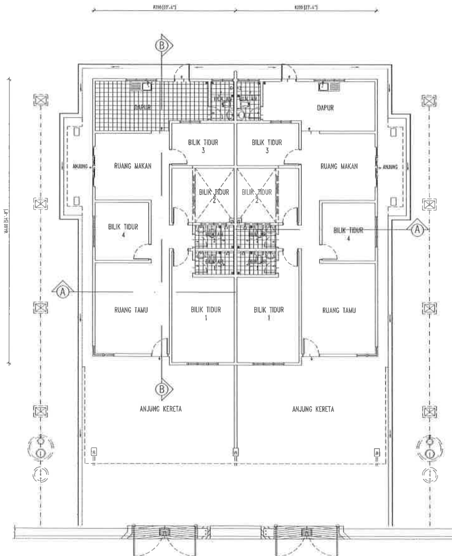
PELAN LANTAI
