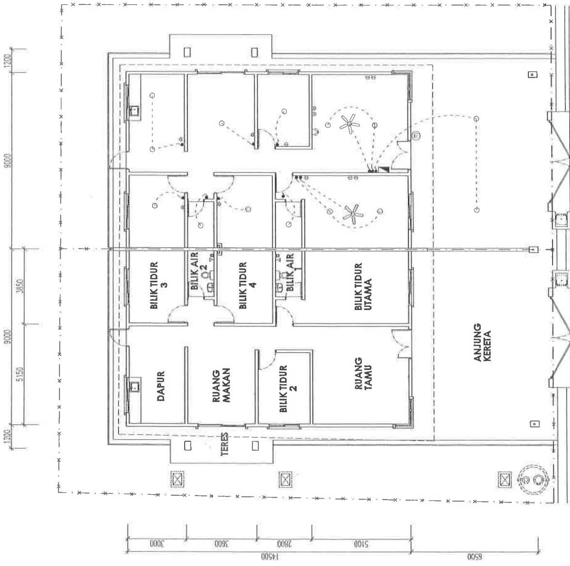
PELAN LANTAI
