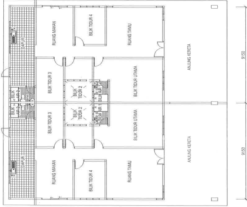
PELAN LANTAI JENIS B
