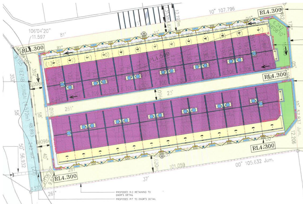
PELAN TAPAK
