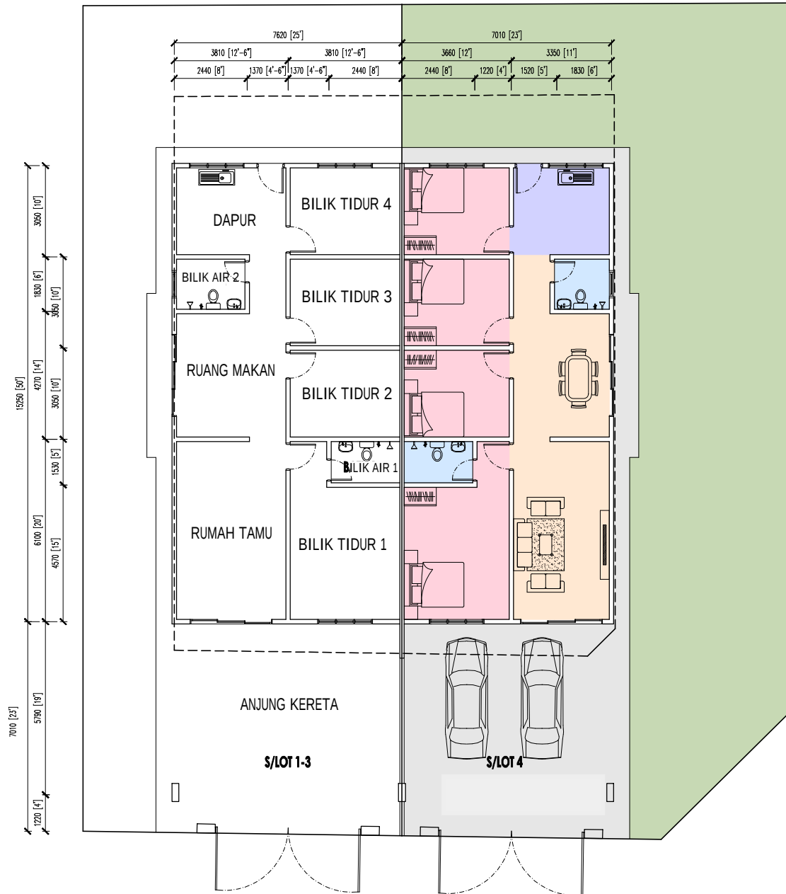
PELAN LANTAI
