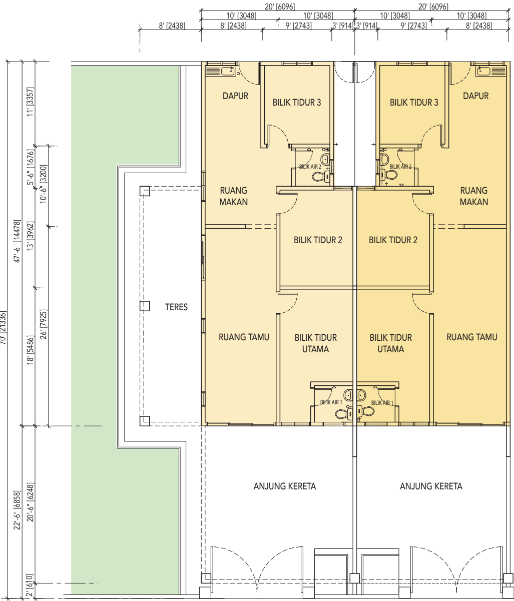
PELAN LANTAI
