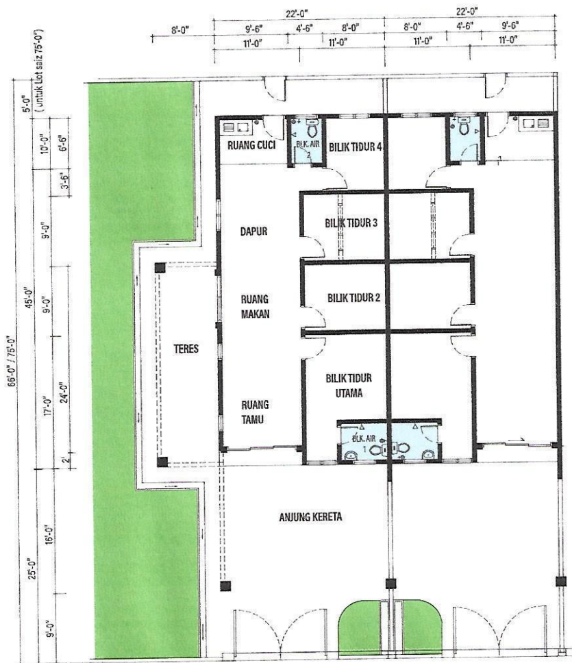
PELAN LANTAI
