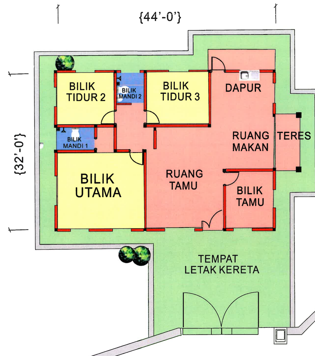
RUMAH BANGLO 1 TINGKAT PELAN LANTAI (32' X 44')
