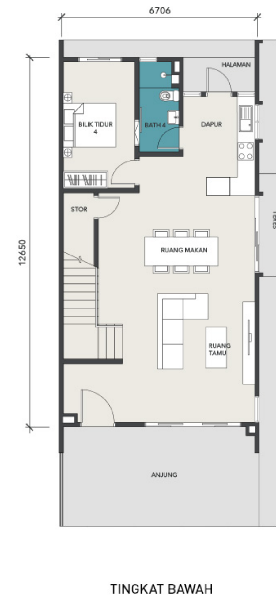
Jenis C 1
