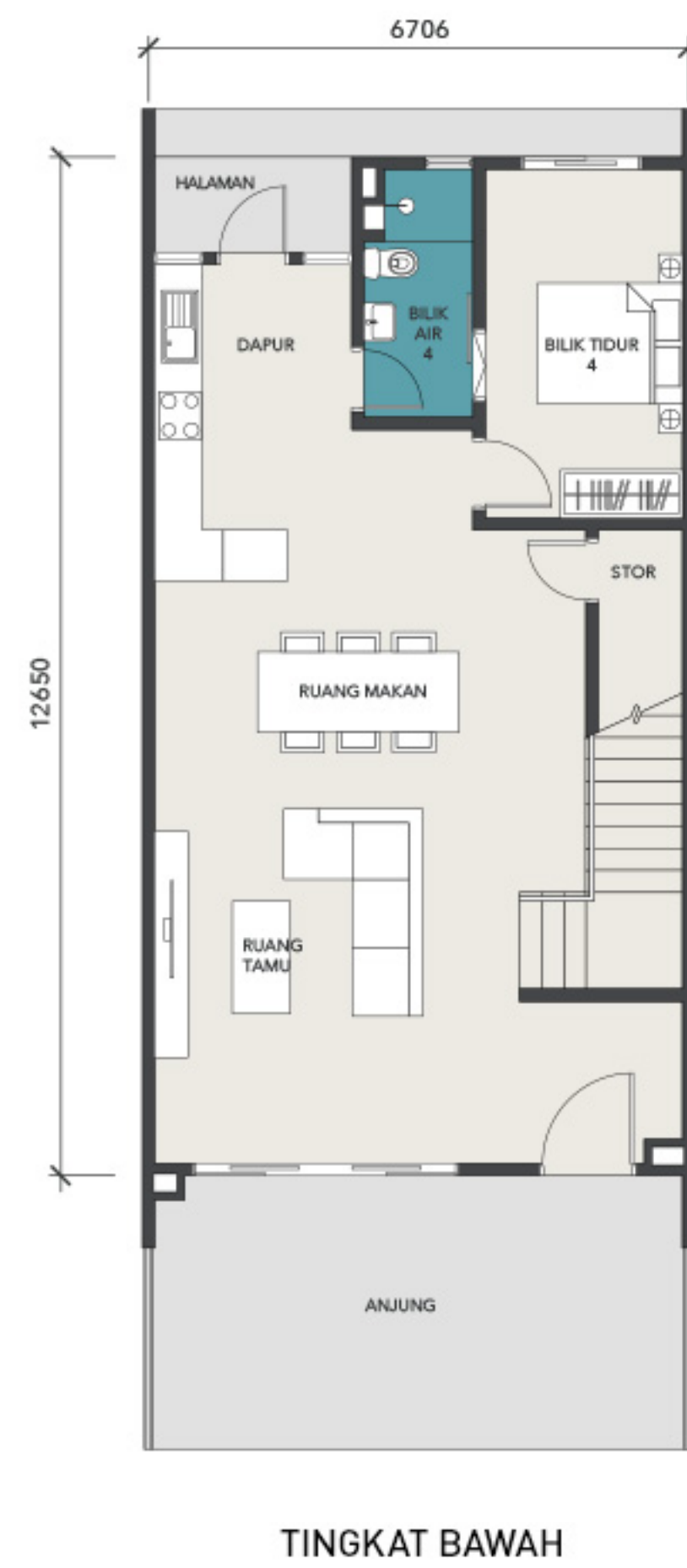
Jenis A 1
