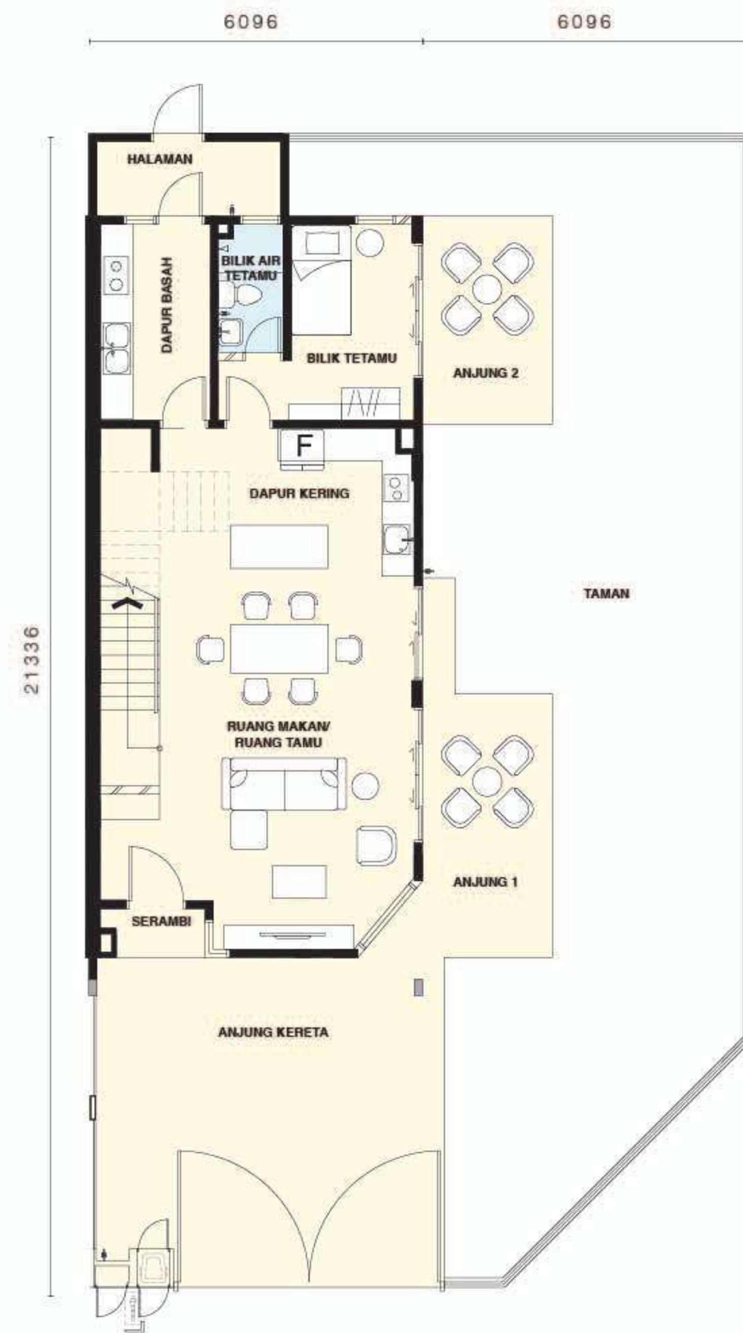
TINGKAT BAWAH
