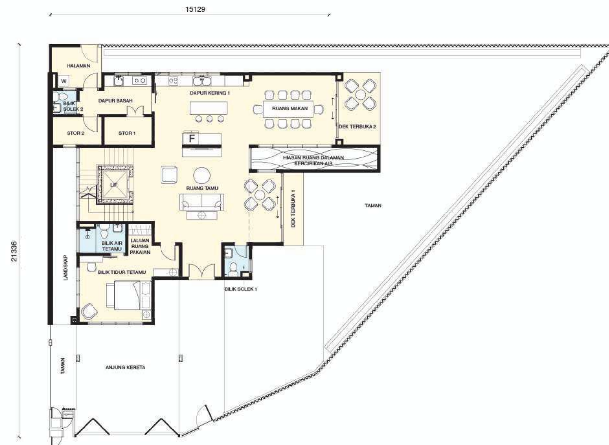
TINGKAT BAWAH
