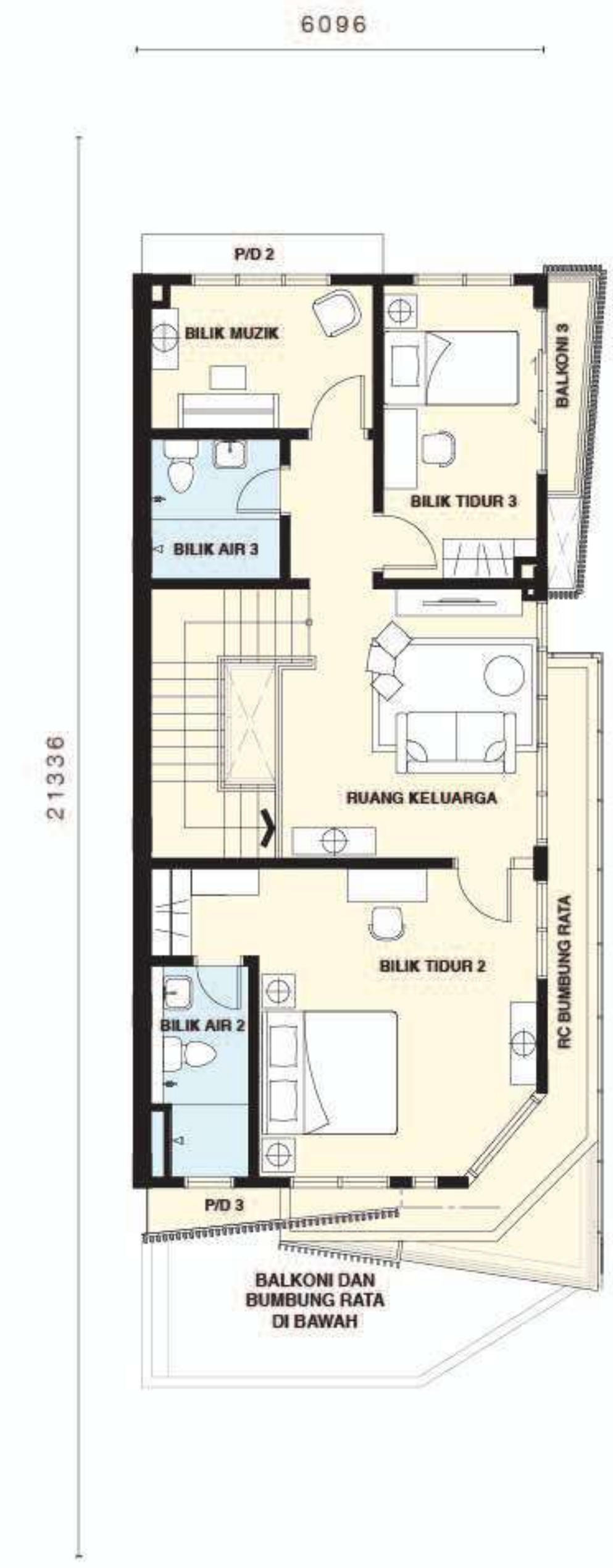
TINGKAT DUA
