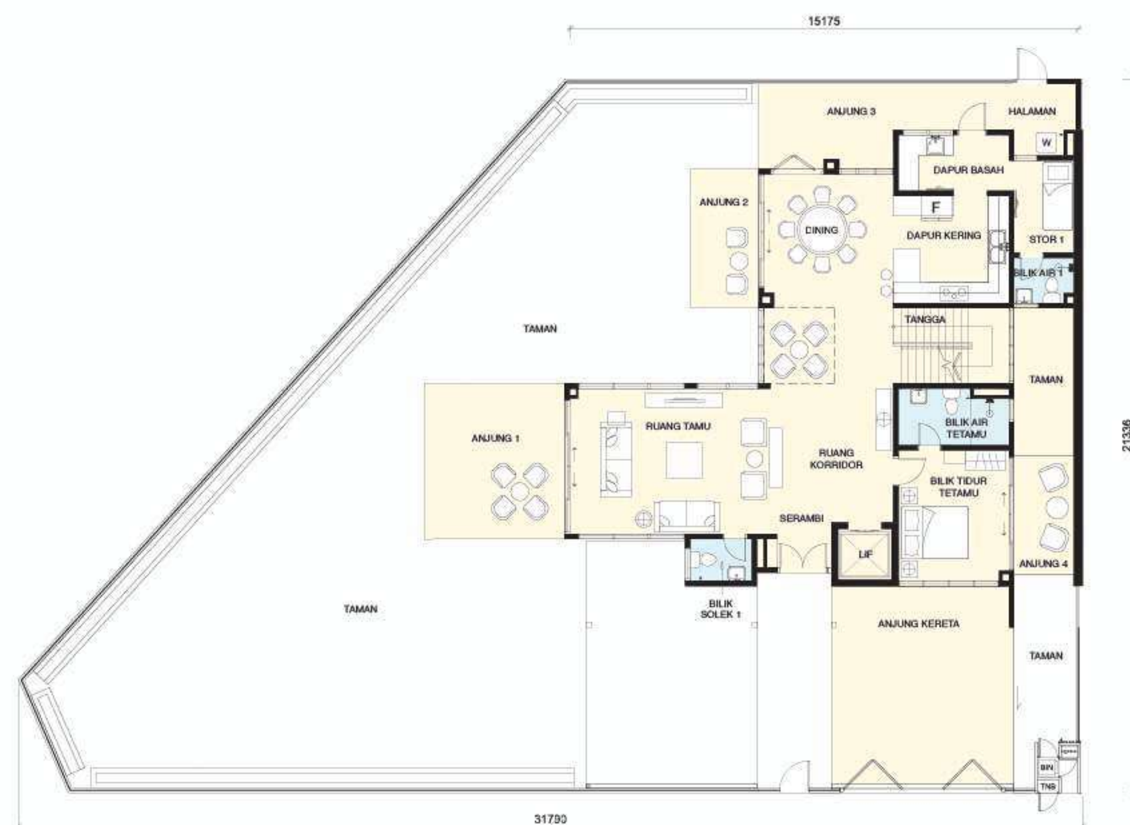
TINGKAT BAWAH
