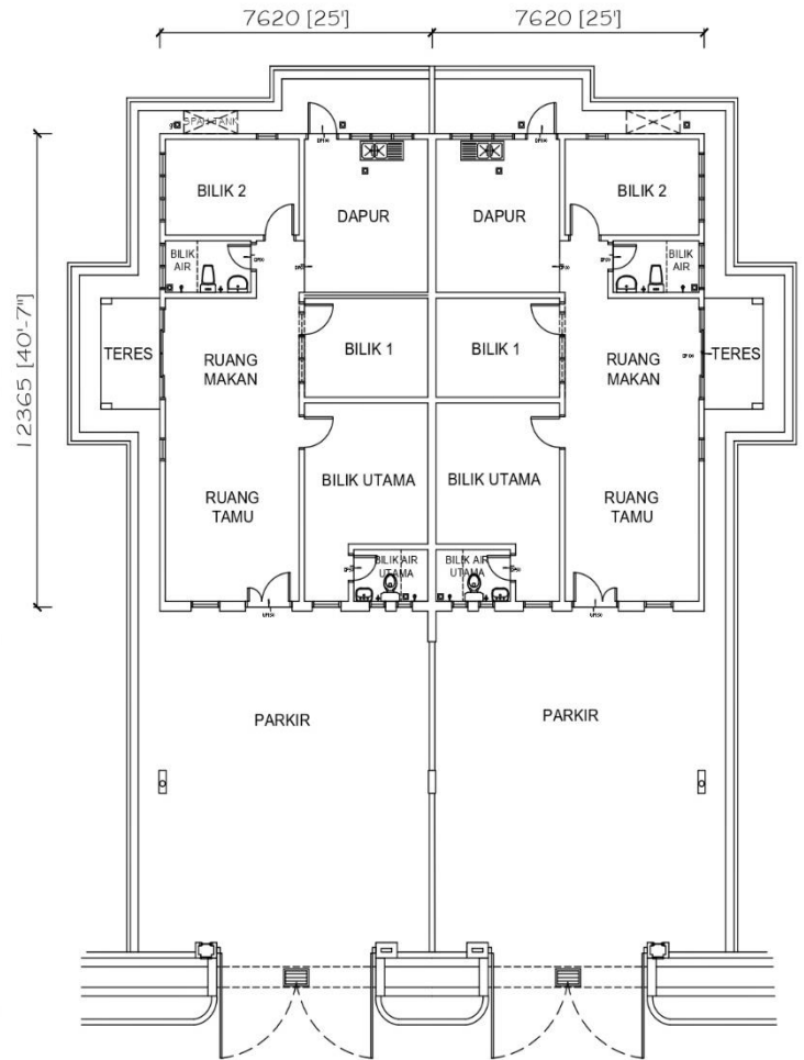
Pelan Lantai
