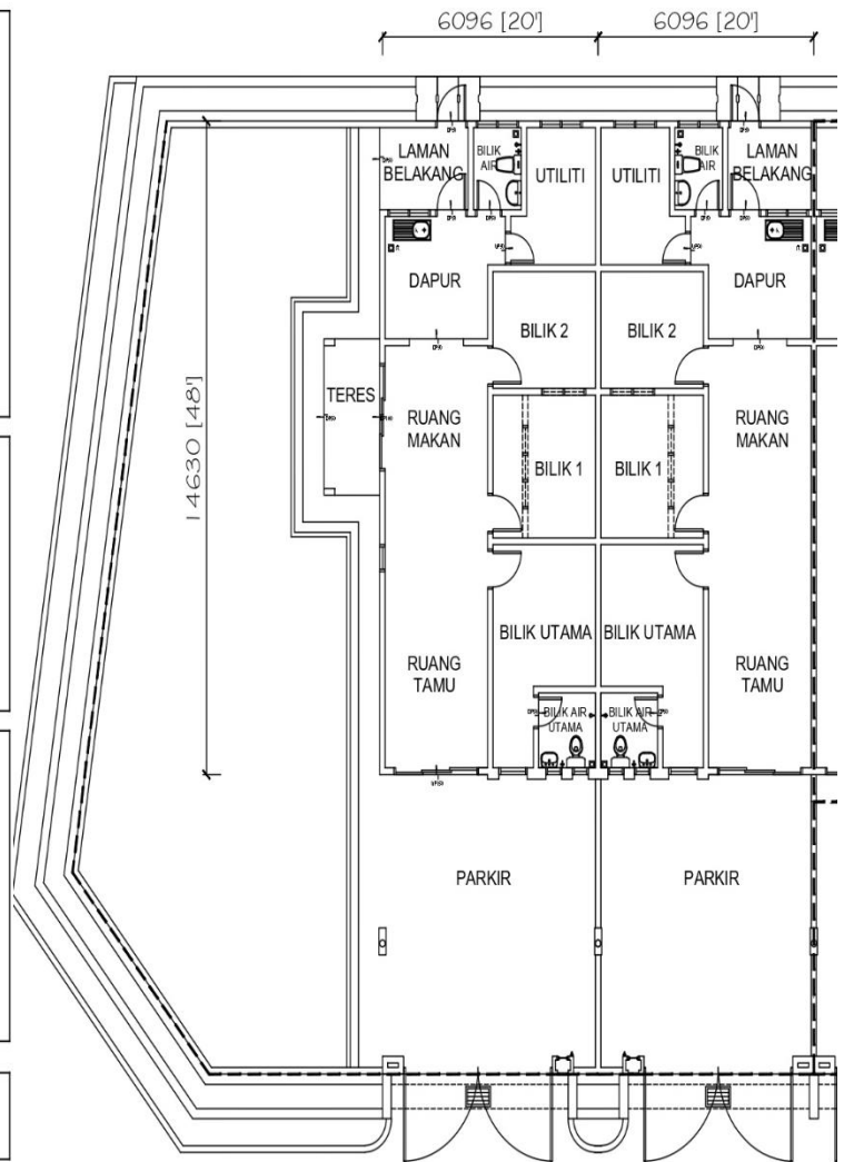
Pelan Lantai
