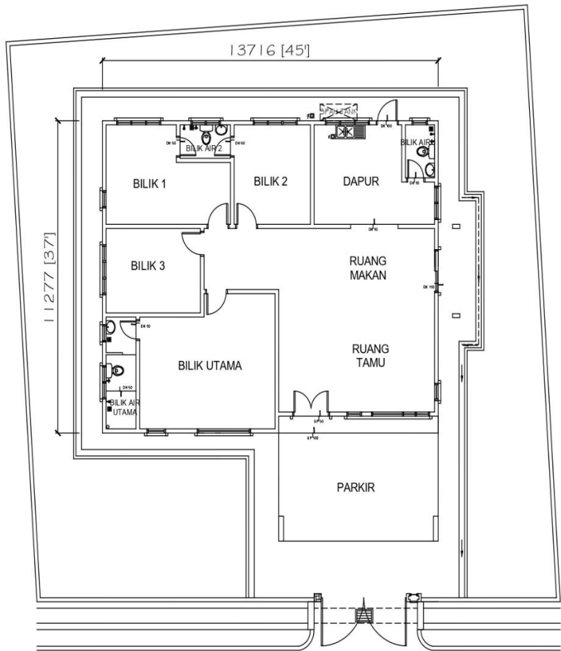
Pelan Lantai
