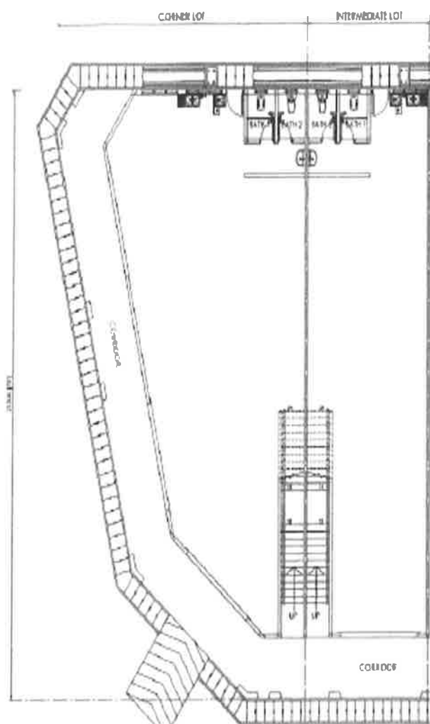
PELAN LANTAI
