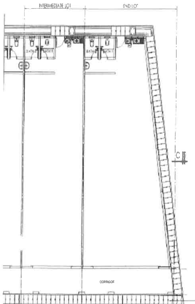
PELAN LANTAI
