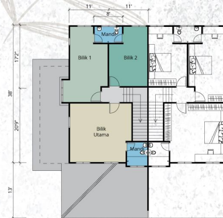
Pelan Tingkat Atas
