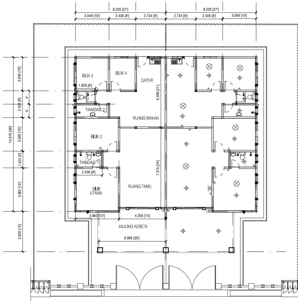
PELAN LANTAI
