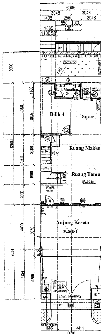
Tingkat Bawah
