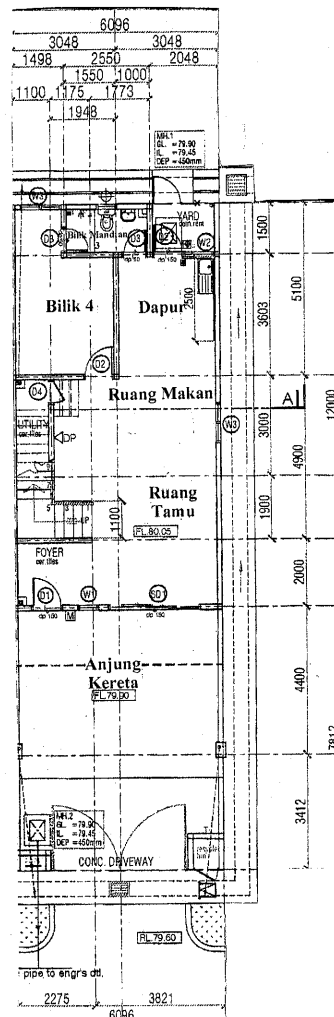
Tingkat Bawah
