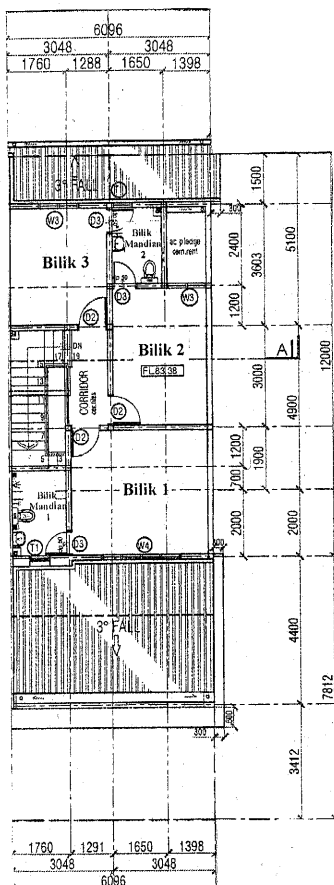
Tingkat Atas
