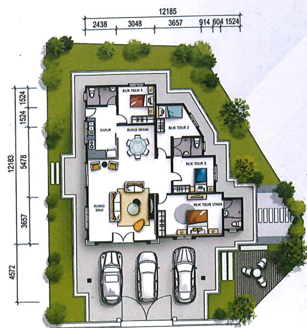
PELAN LANTAI RUMAH BANGLO SETINGKAT - JENIS B
