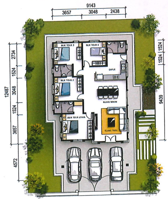
PELAN LANTAI RUMAH BANGLO SETINGKAT - JENIS A
