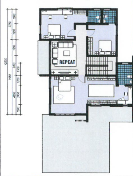
12 Unit Rumah Teres Setingkat (Baki 6 unit)
