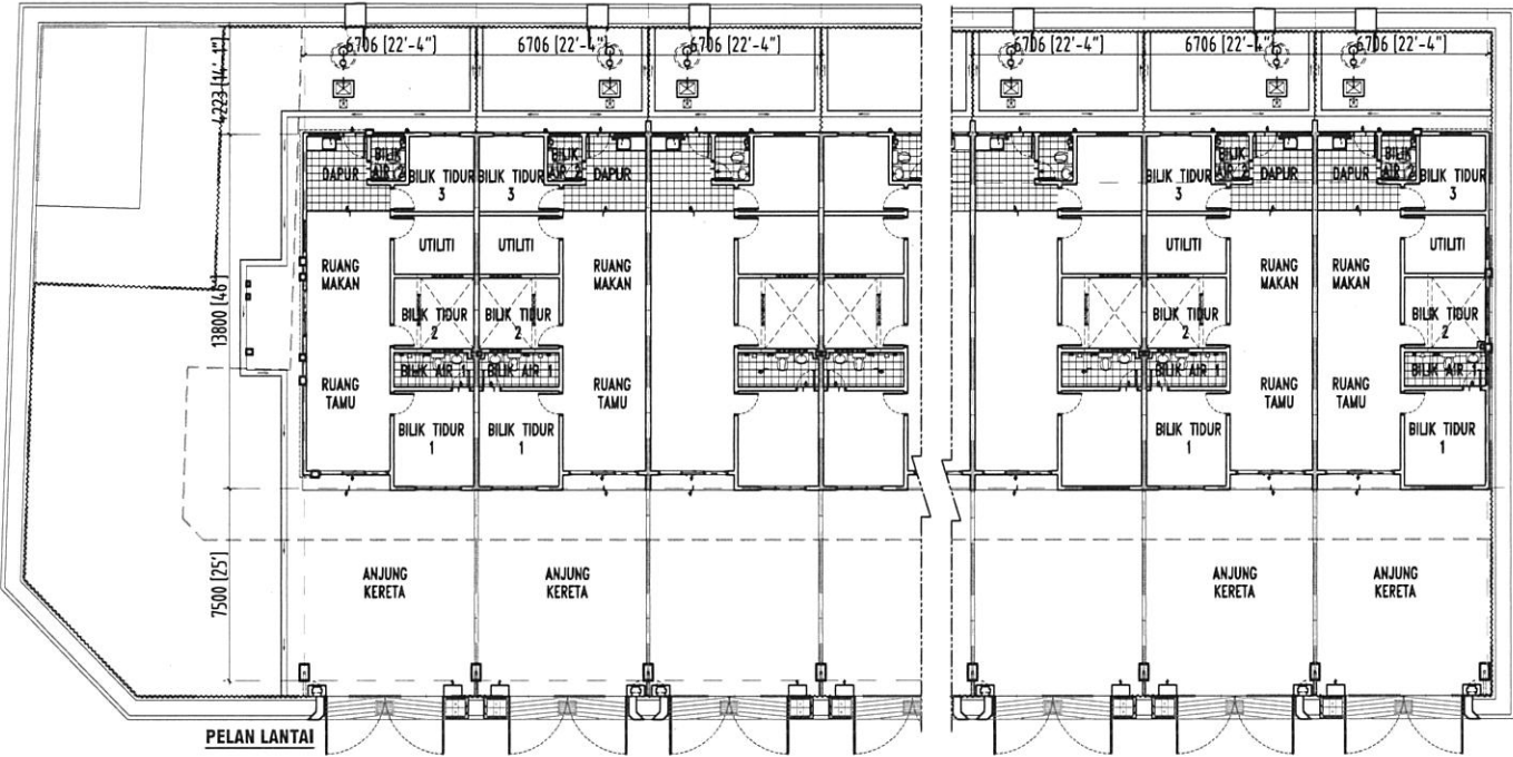
PELAN LANTAI
