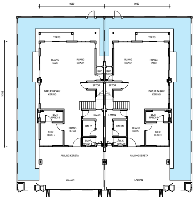
PELAN ARAS BAWAH
