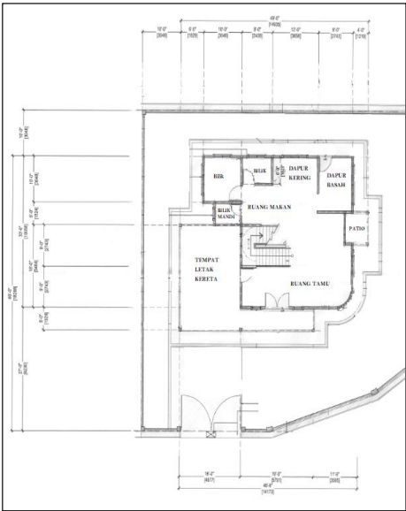
TINGKAT BAWAH
