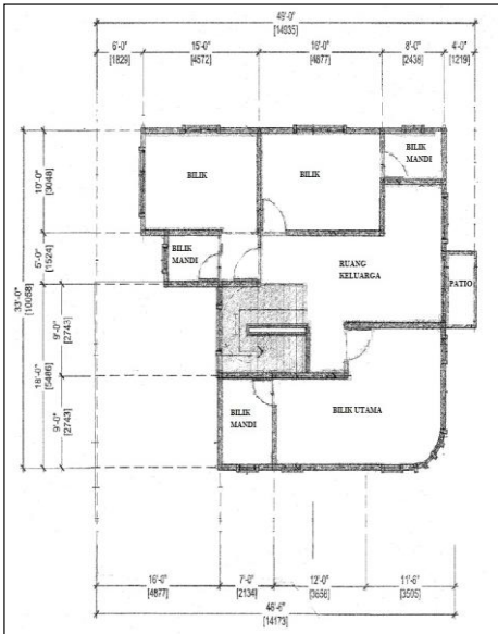
TINGKAT ATAS
