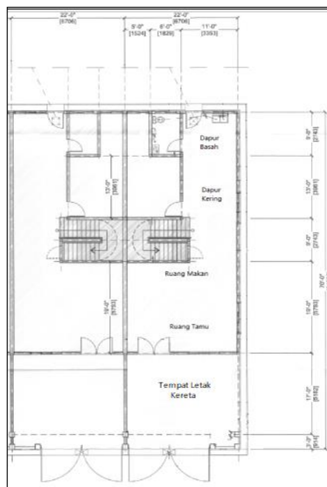
TINGKAT BAWAH
