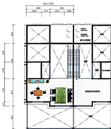
TINGKAT MEZANIN
