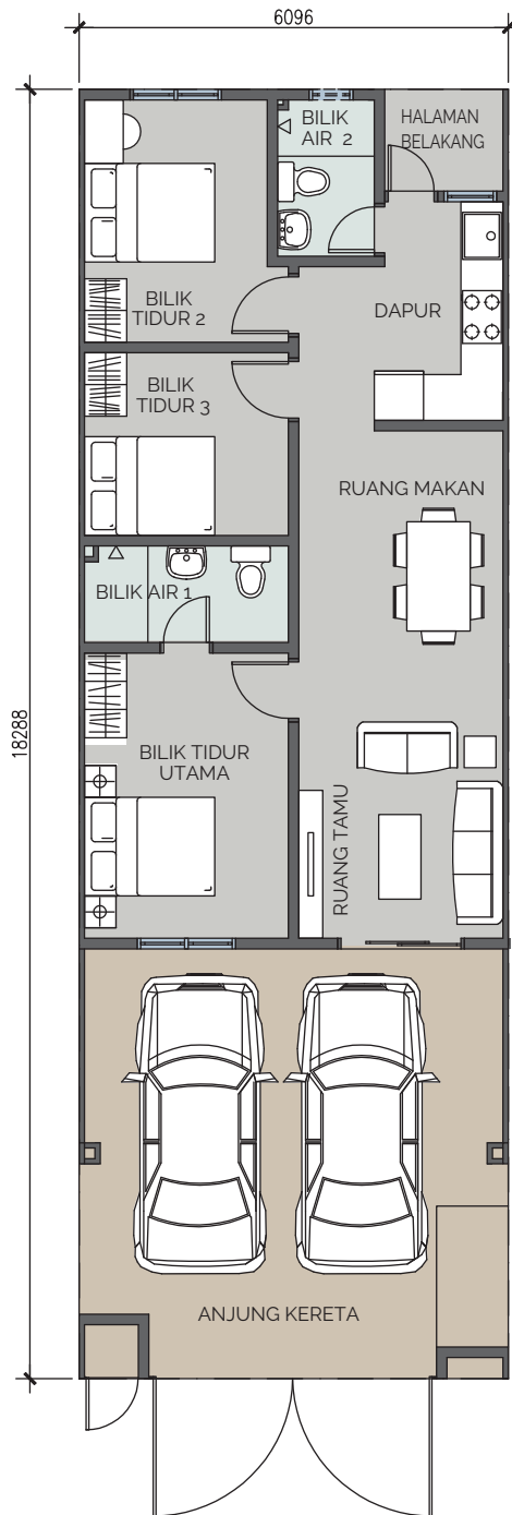
Pelan Tingkat Bawah (Lot Tengah)
