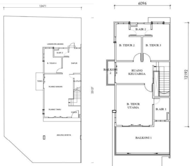
Pelan Lantai Tipikal
