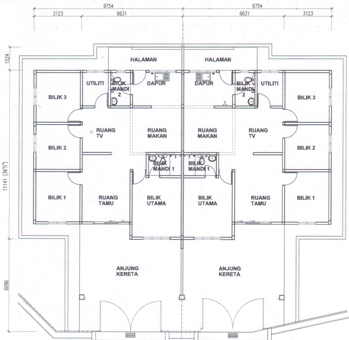
PELAN LANTAI (RUMAH BERKEMBAR 1 TINGKAT)
