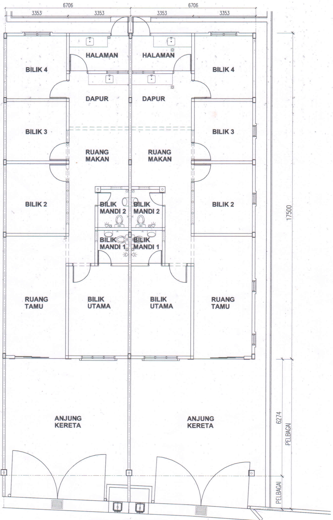
PELAN LANTAI (RUMAH TERES 1 TINGKAT)
