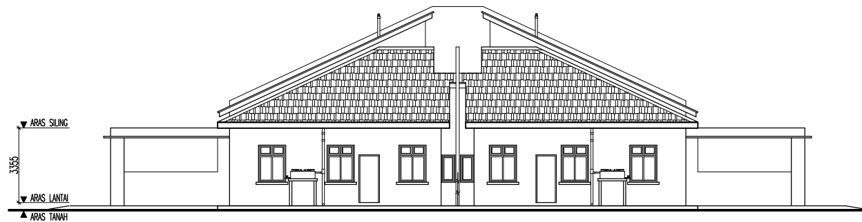
PANDANGAN SISI
