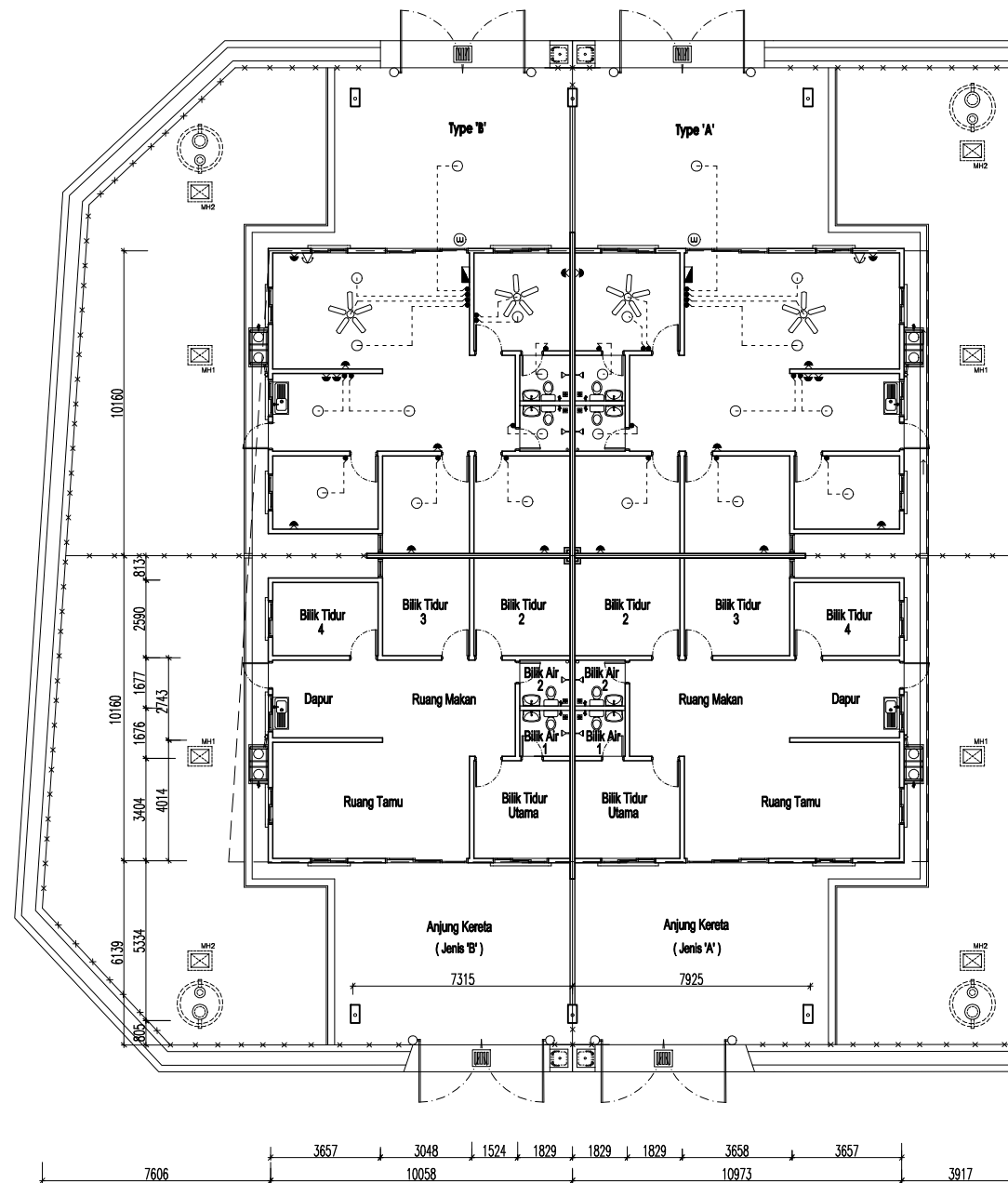
PELAN LANTAI
