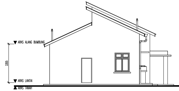
PANDANGAN BELAKANG
