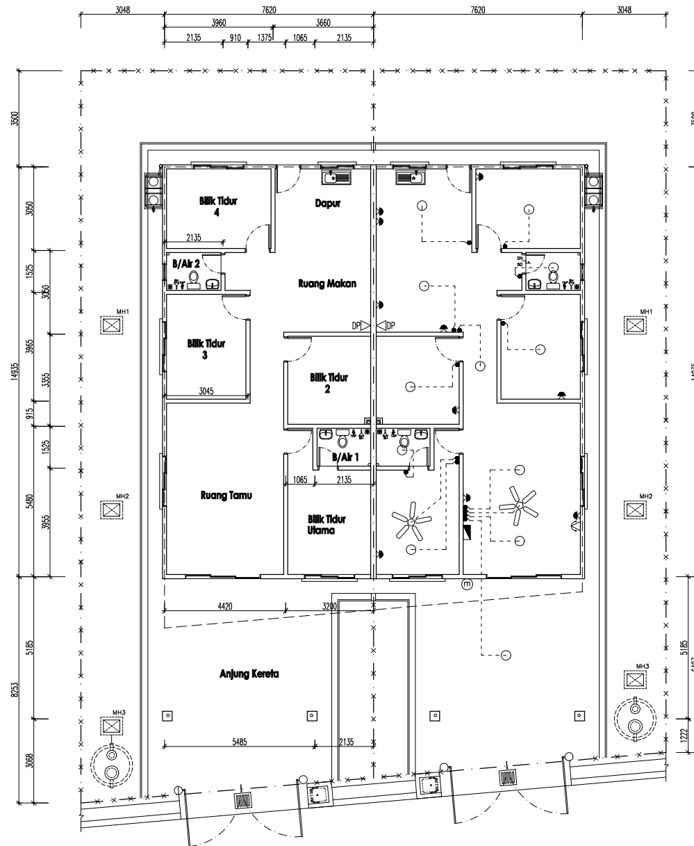
PELAN LANTAI
