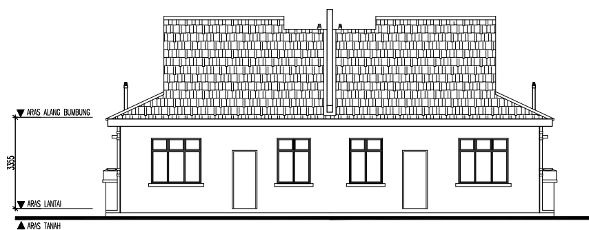
PANDANGAN BELAKANG
