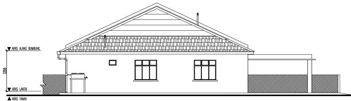
PANDANGAN SISI
