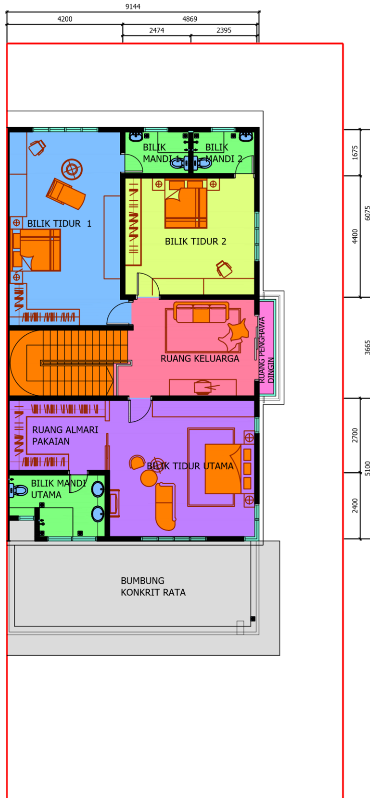
PELAN LANTAI TINGKAT SATU
