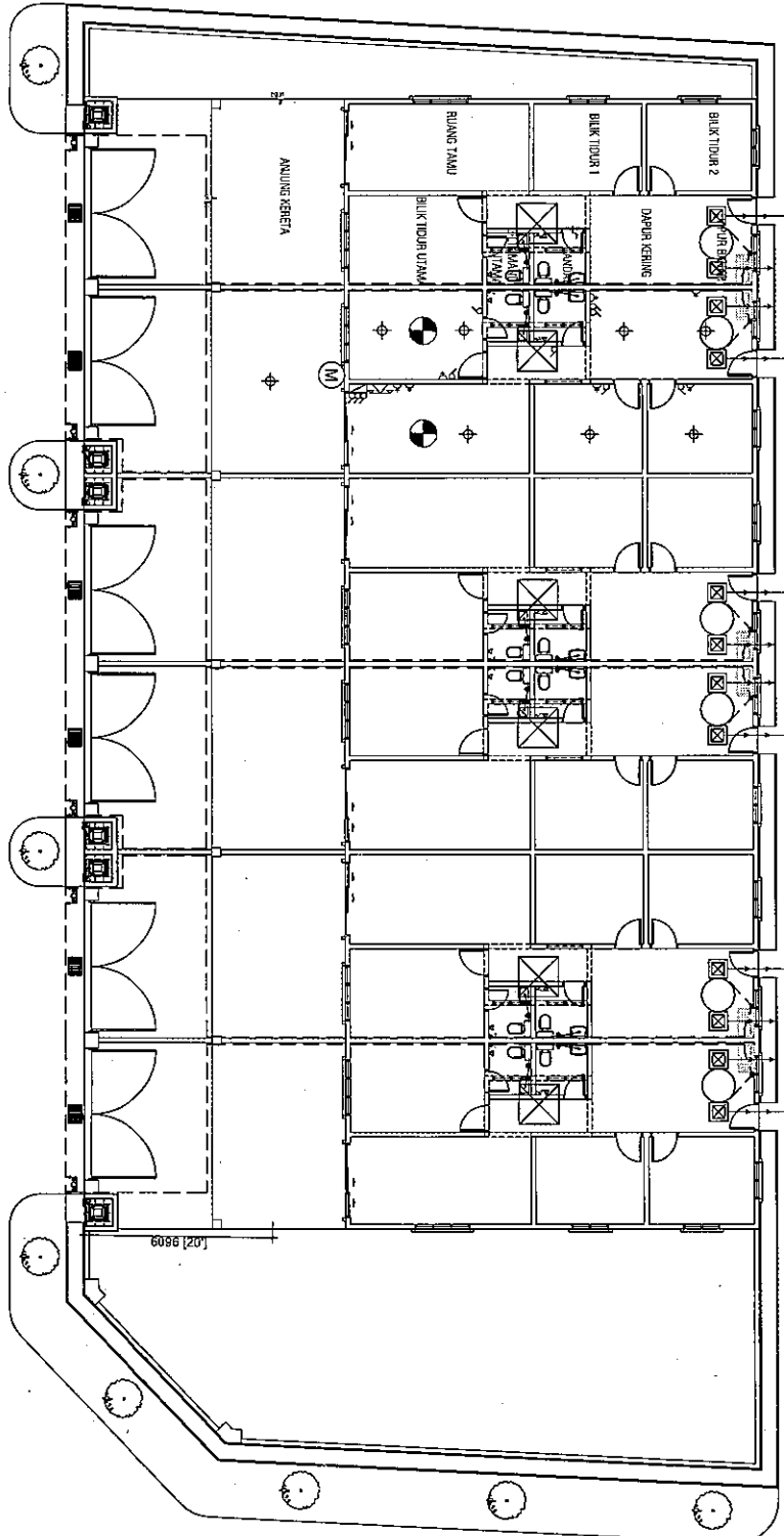
PELAN LANTAI JENIS "A"
