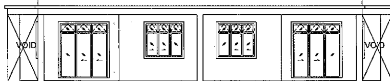
PANDANGAN DEPAN RUMAH BERBANDUNG (PTD. 16155 & 16156)
