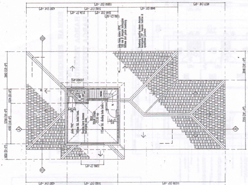
PELAN LANTAI TINGKAT SATU DAN BUMBUNG
