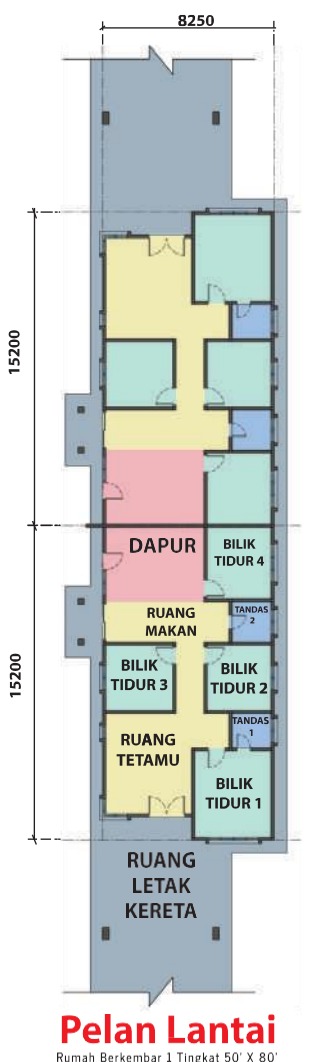
Pelan Lantai
