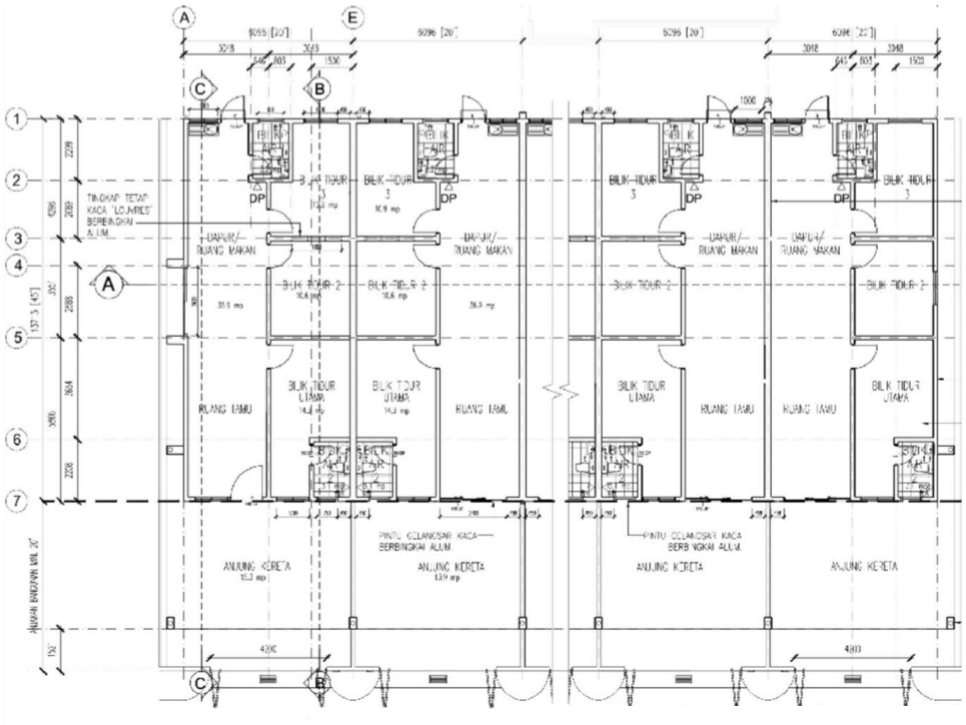
PELAN LANTAI TINGKAT BAWAH (TERES JENIS A)
