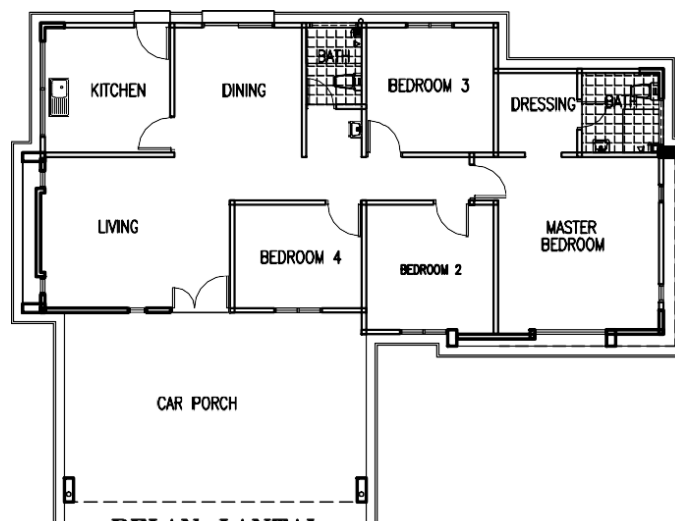
PELAN LANTAI
