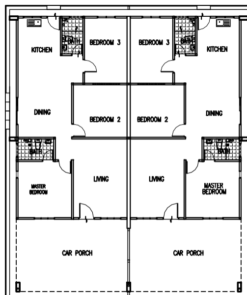
PELAN LANTAI
