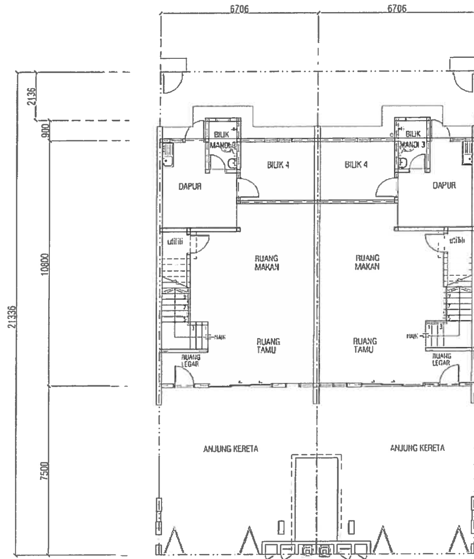
Pelan Lantai - Tingkat Bawah
