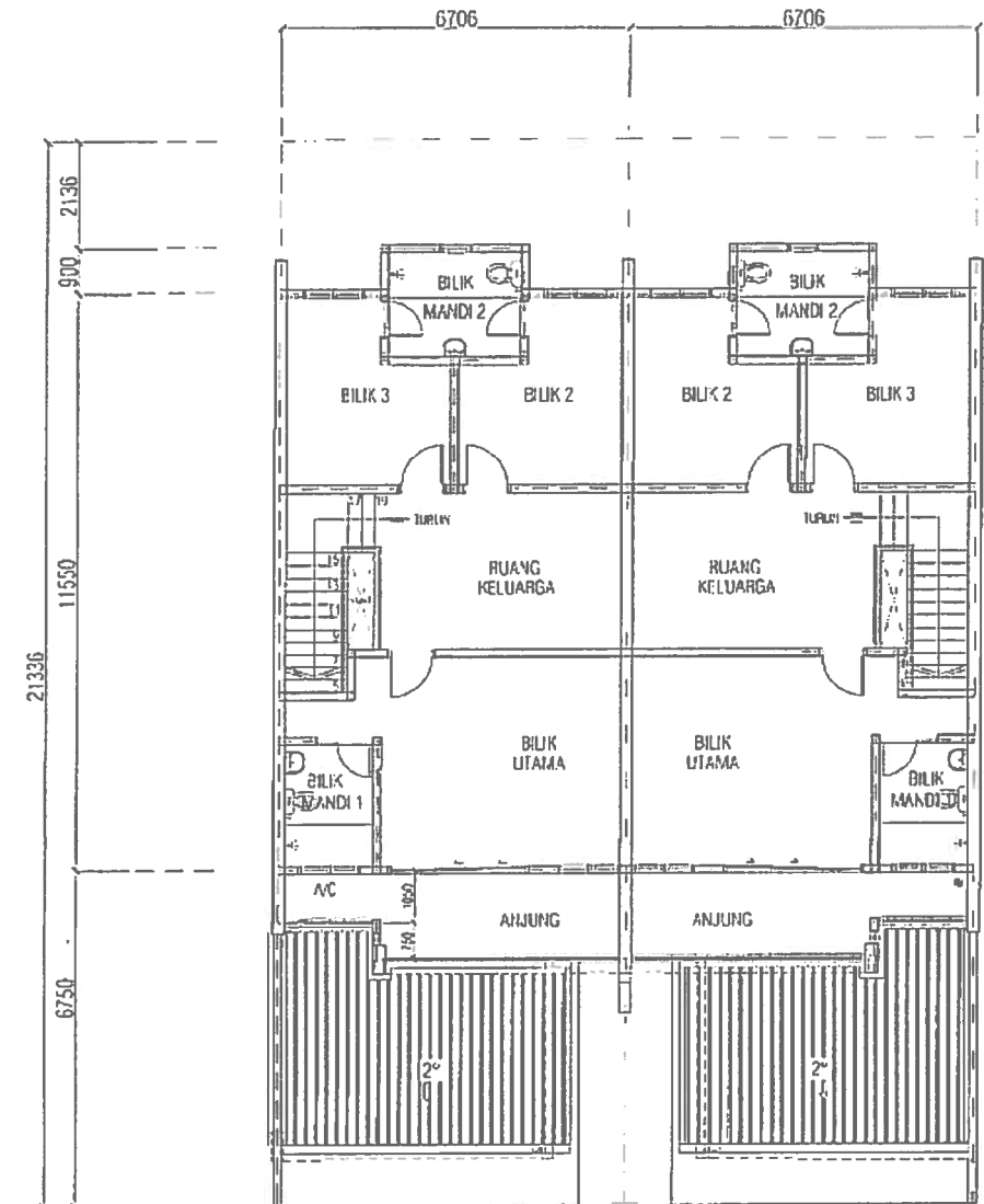
Pelan Lantai - Tingkat 1
