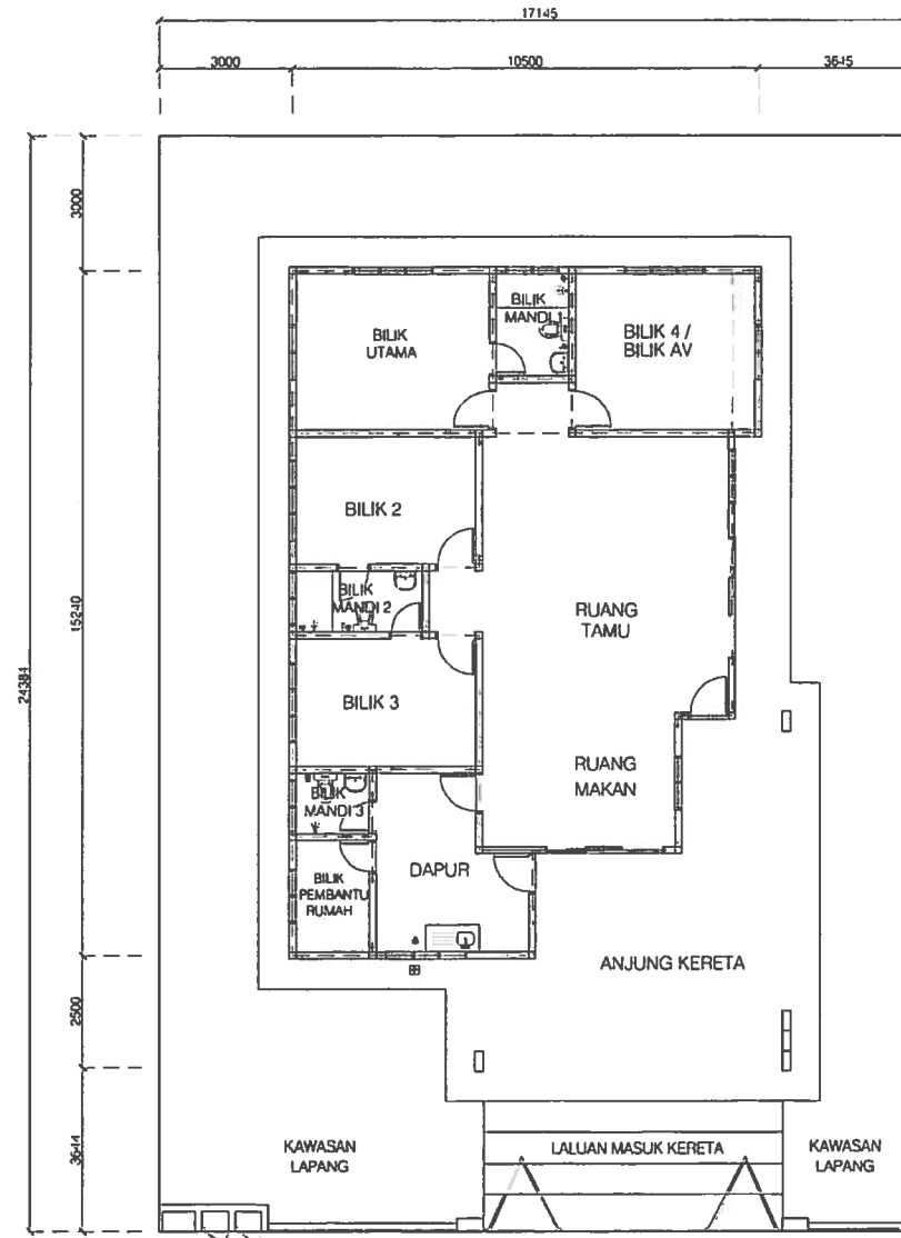
Pelan Lantai Tipikal
