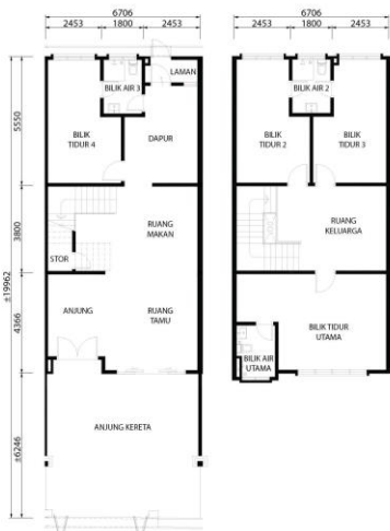
Pelan Lantai
