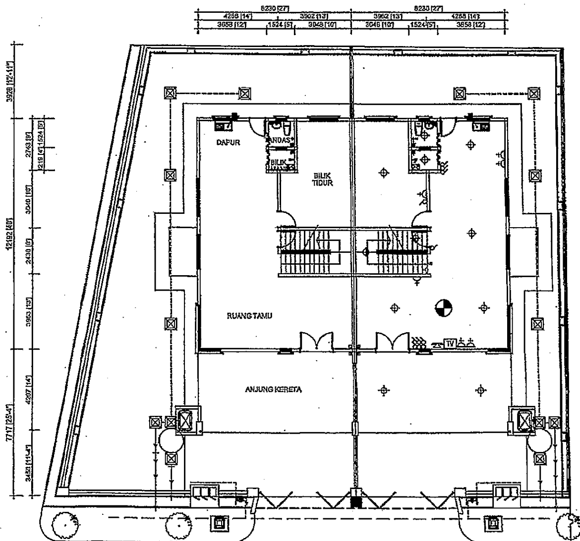
PELAN LANTAI
