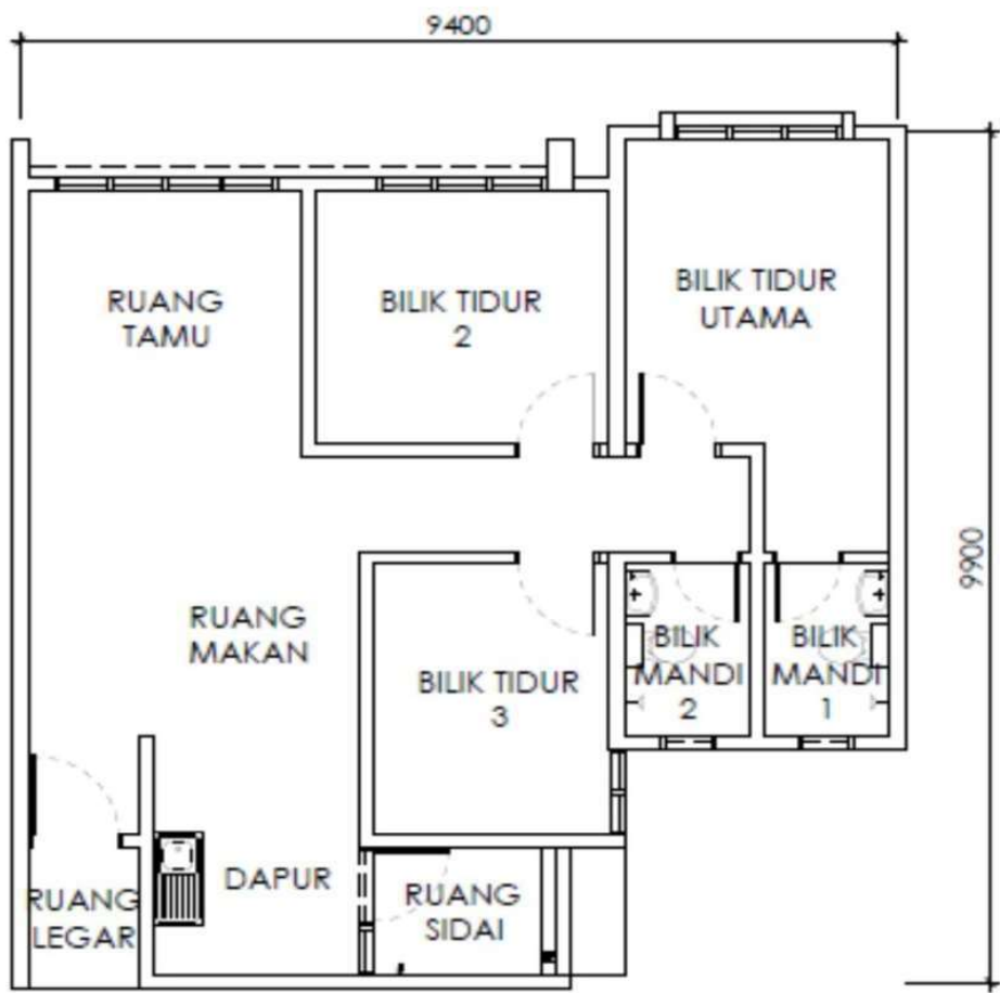
Pelan Lantai
