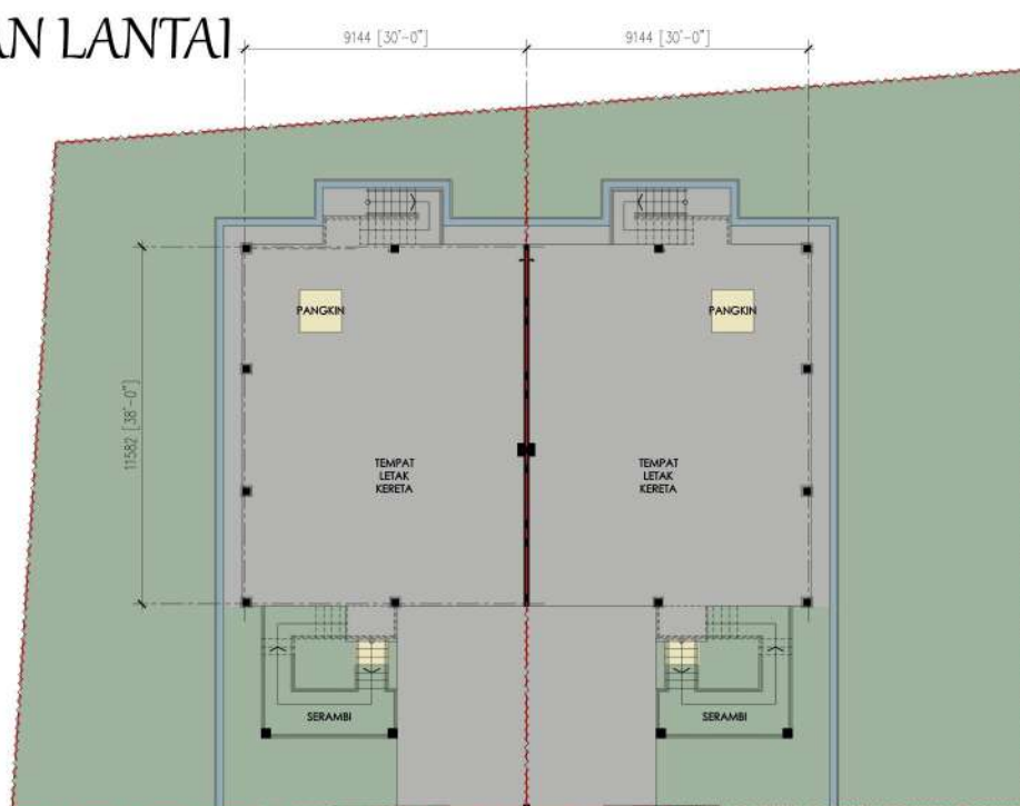
TINGKAT BAWAH
