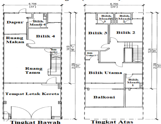
Pelan Lantai
