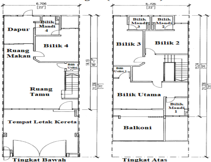
Rumah Teres 2 Tingkat (Jenis 1 : A1) - 22' x 70'
