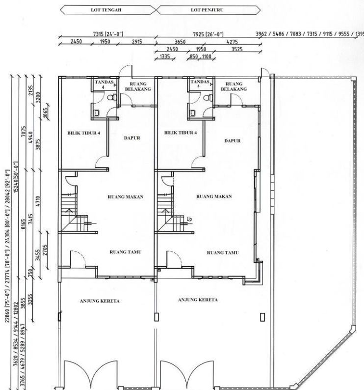
Pelan Tingkat Bawah (楼下平面图)
