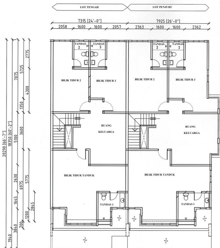
Pelan Tingkat Atas (楼上平面图)
