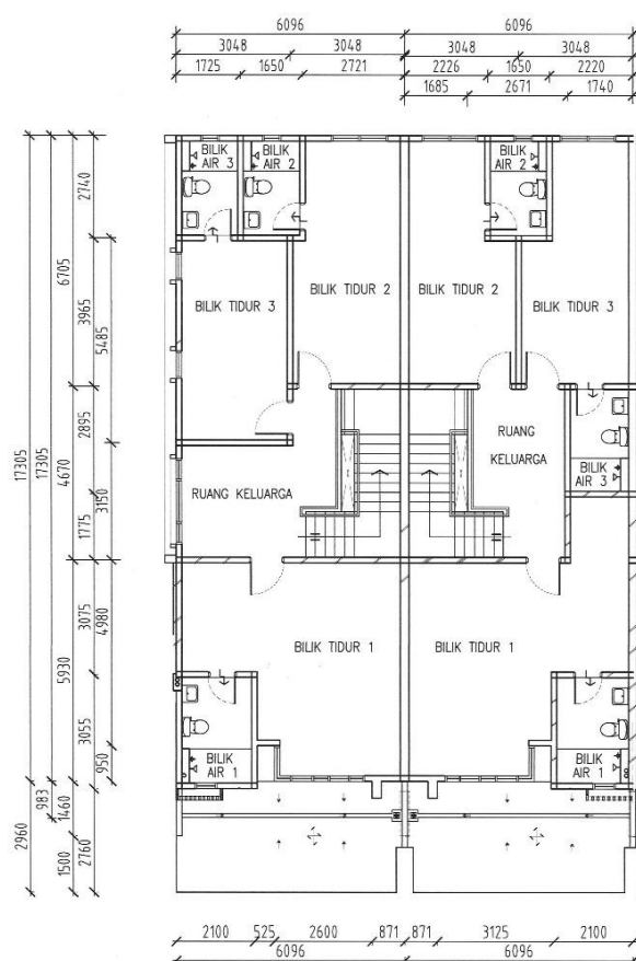
Pelan Tingkat Satu
