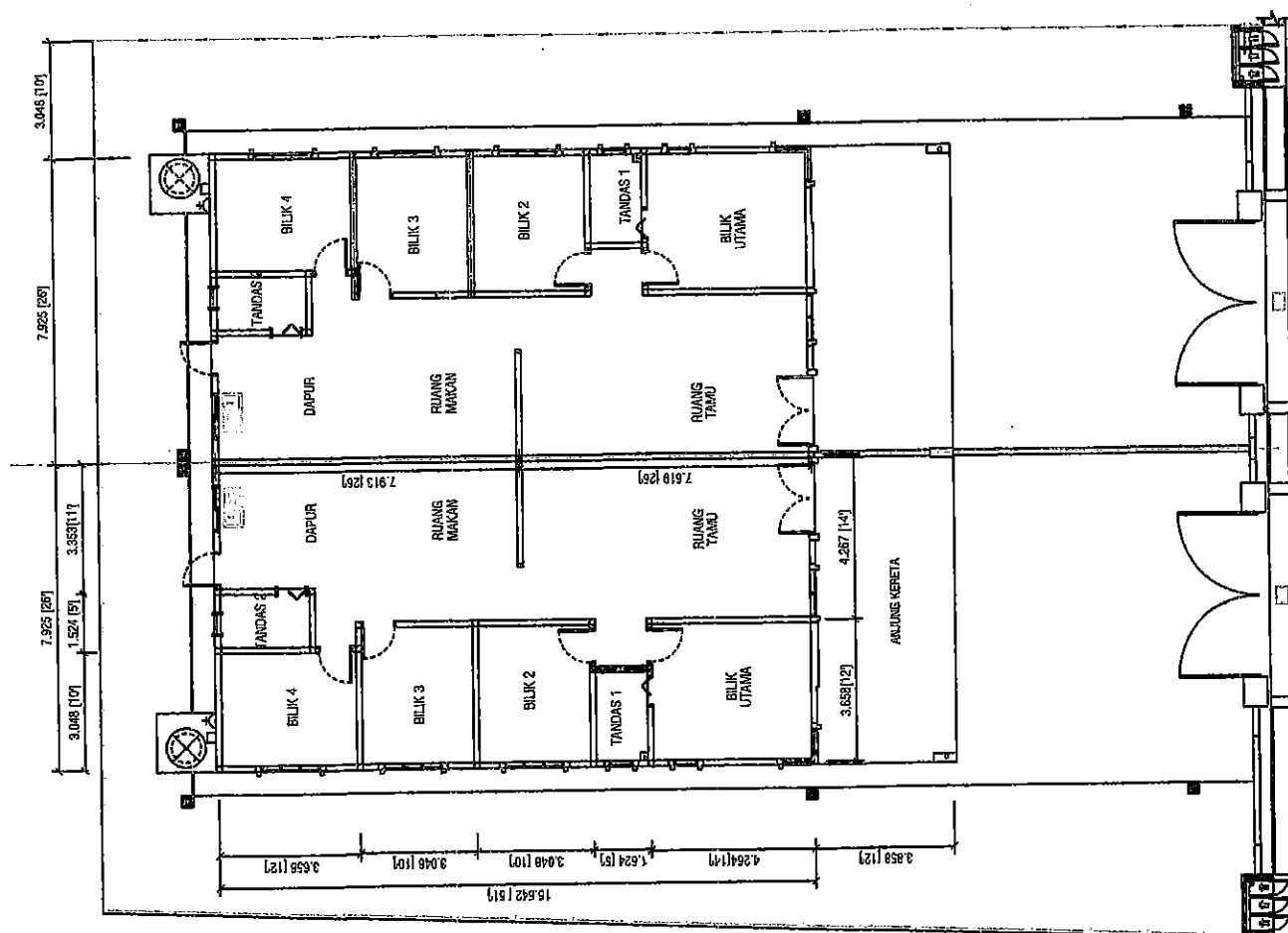
PELAN LANTAI RUMAH BERBANGUNG SATU TINGKAT - (PTD 8041-PTD 8044)
