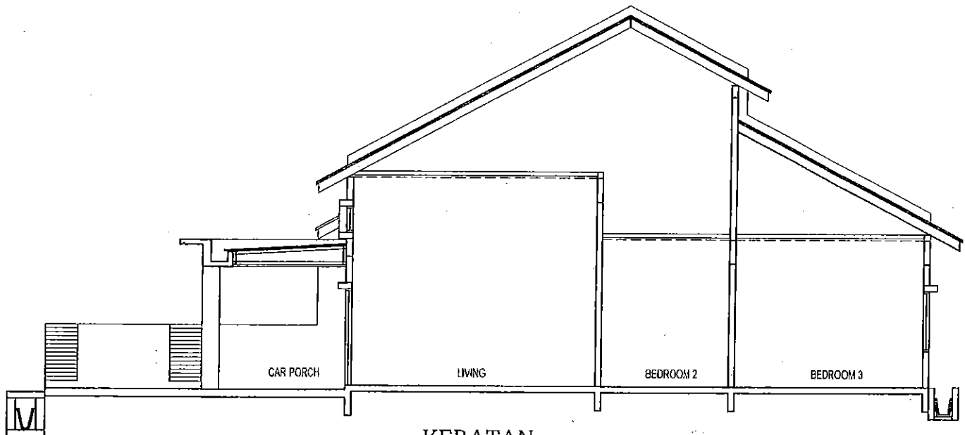
KERATAN
