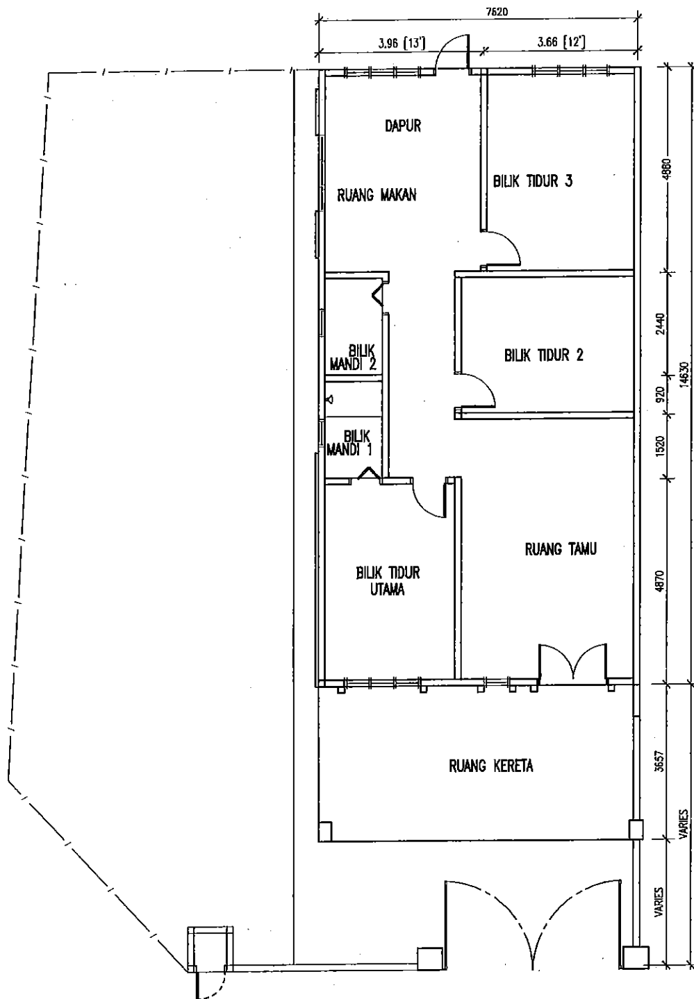
PELAN LANTAI
