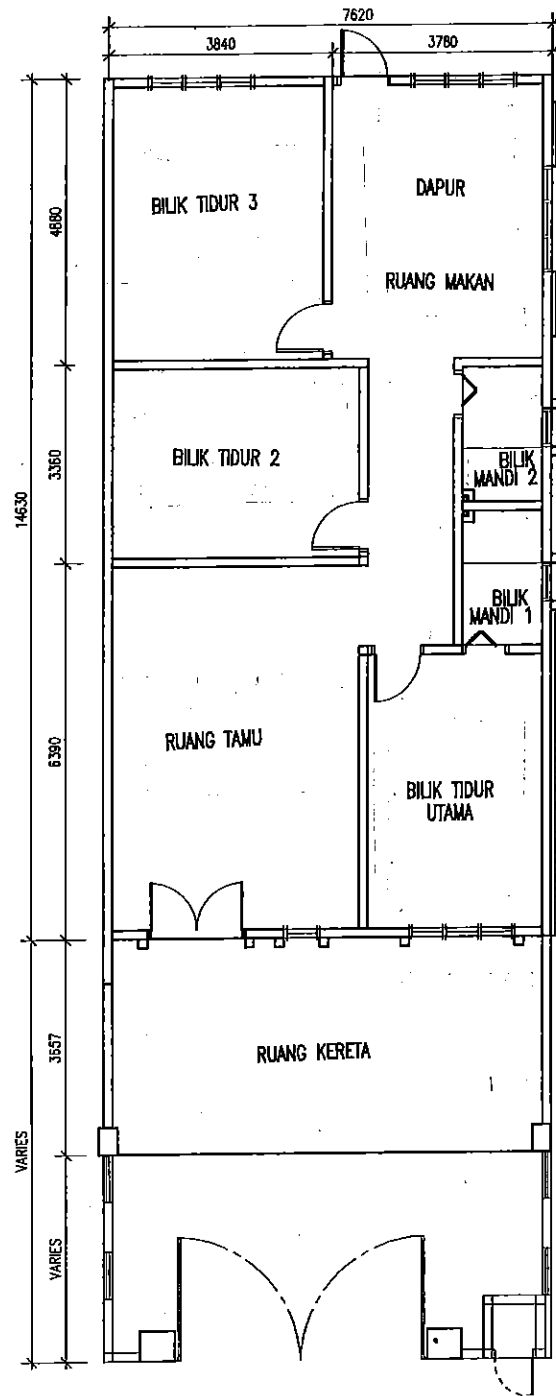
PELAN LANTAI
