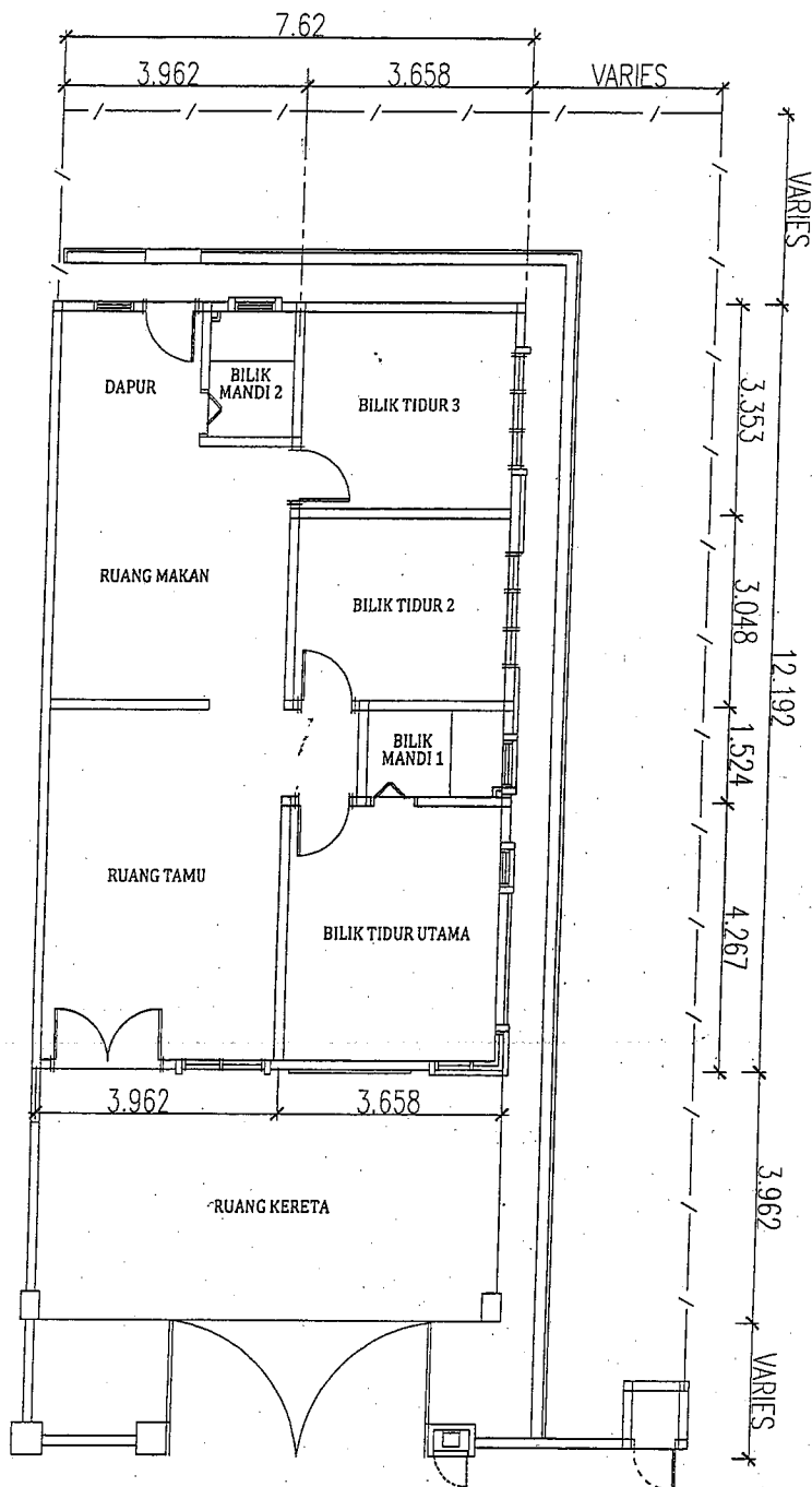
PELAN LANTAI
