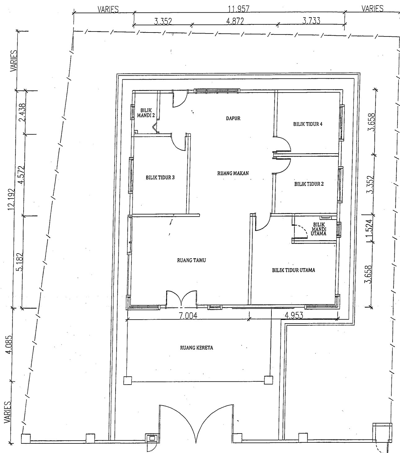
PELAN LANTAI
