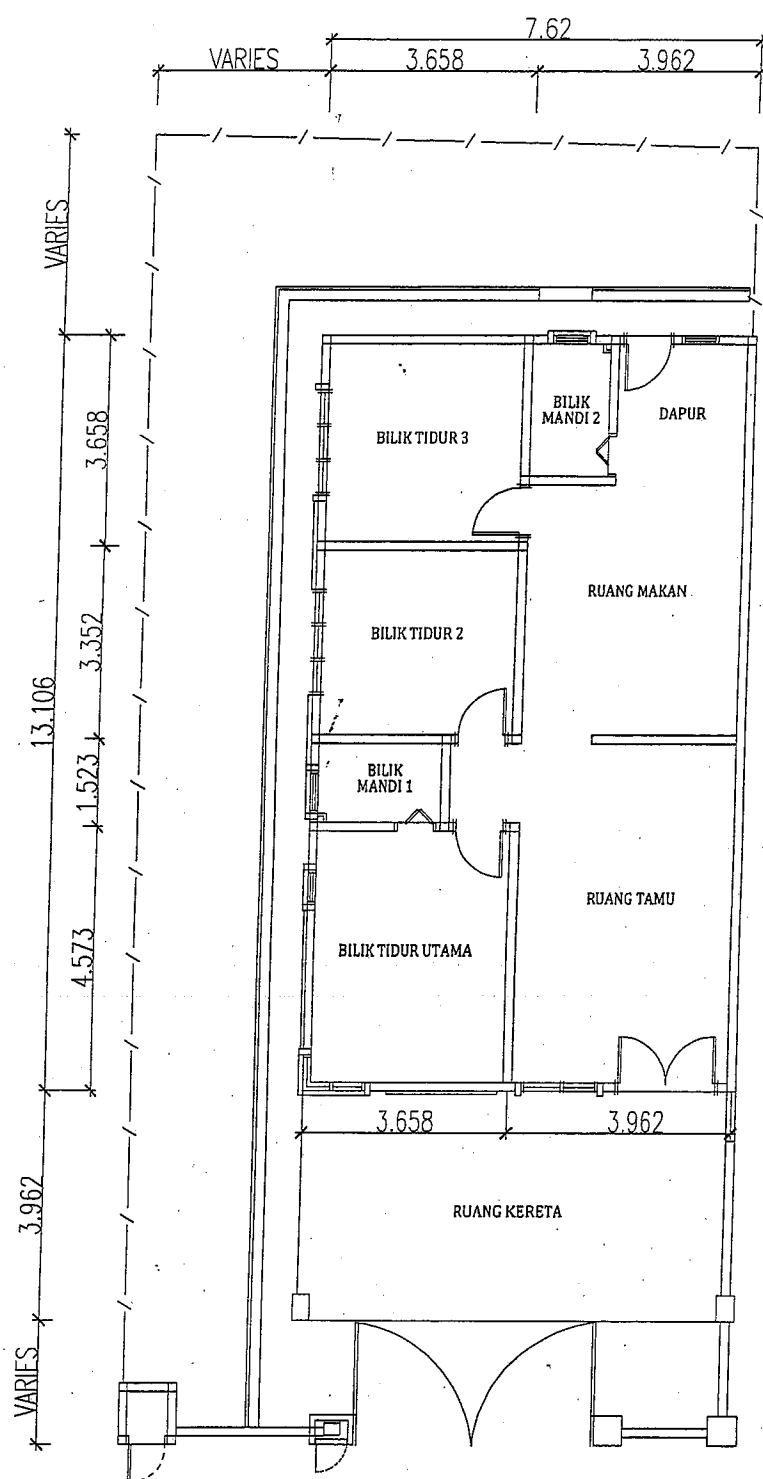
PELAN LANTAI
