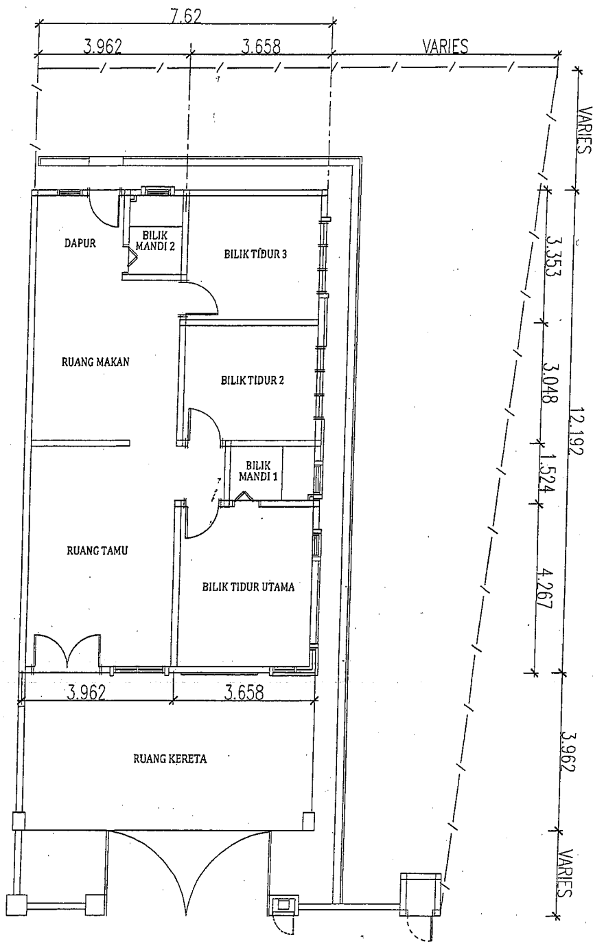
PELAN LANTAI
