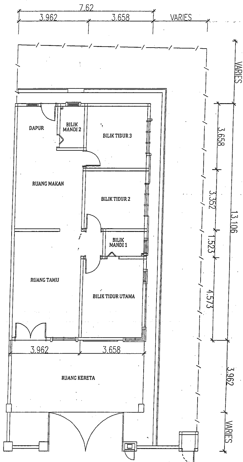
PELAN LANTAI
