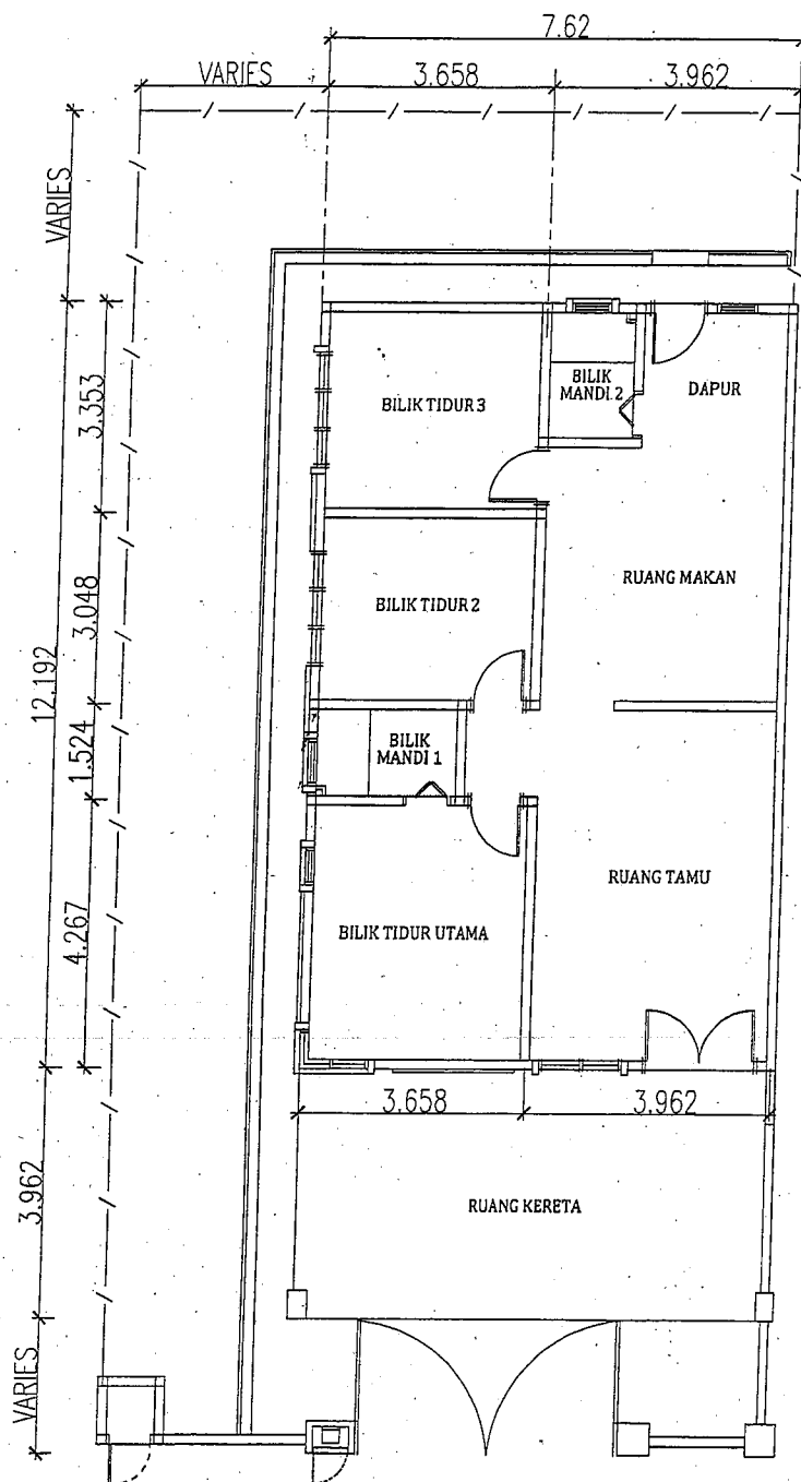
PELAN LANTAI
