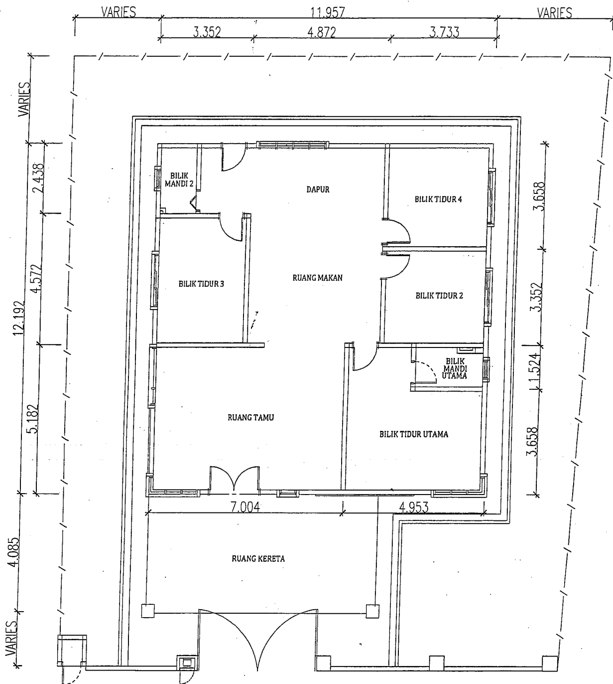
PELAN LANTAI
