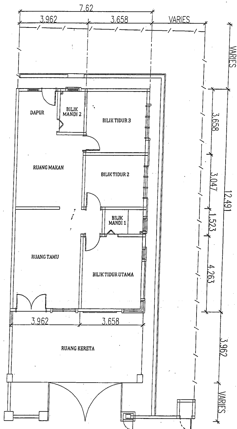
PELAN LANTAI
