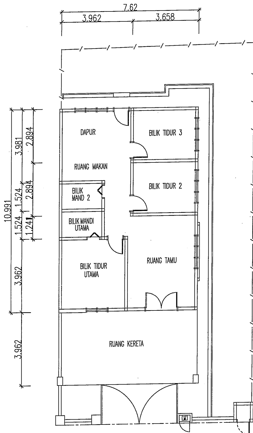
PELAN
