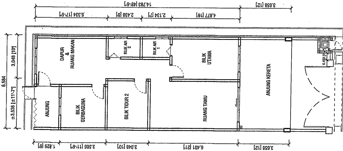
PELAN LANTAI PTD 24733
