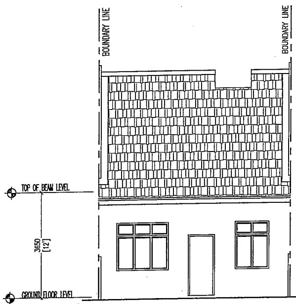
PANDANGAN BELAKANG
